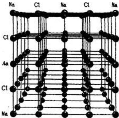
Рис. 1. Кристаллическая решетка галита
