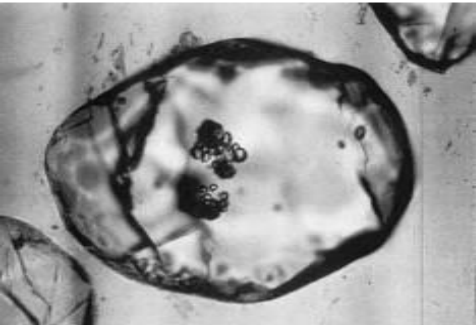
Микроалмазы в кристалле циркона из метаморфических пород (200 микрон по длине, Казахстан )
