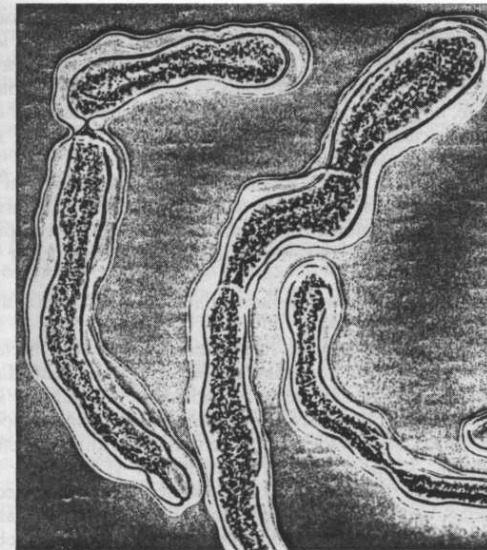
Рис. 5. Простейший биоорганизм Mycoplasma genitalium
