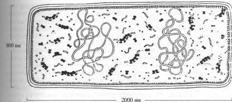
Рис. 6. Бактериальная клетка Echericia coli – мечта нанотехнолога
