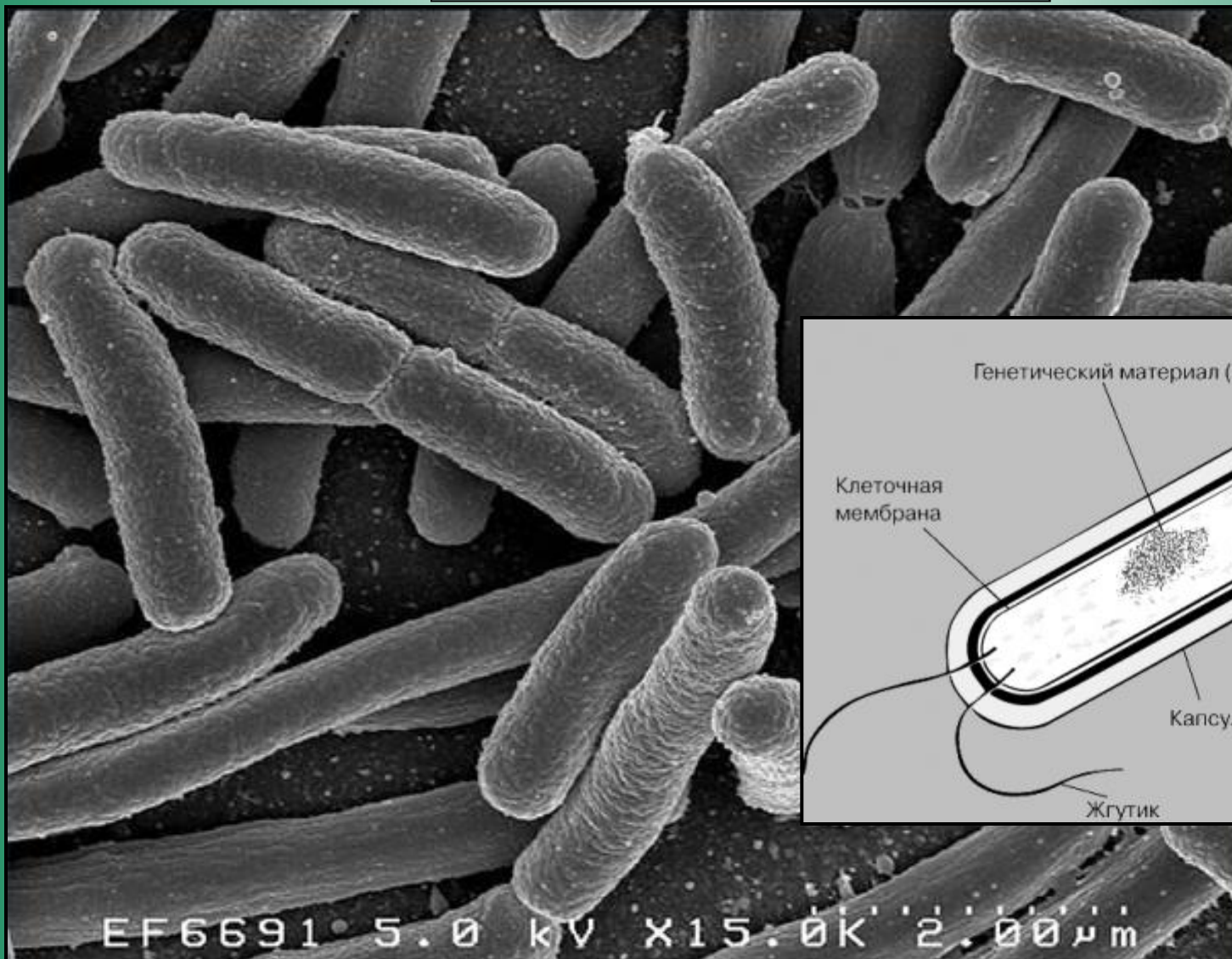
«Типичная бактериальная клетка и ее основные структуры»
