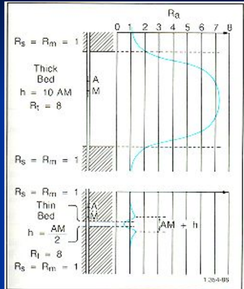
Кривые потенциал-зонда для пластов высокого сопротивления
