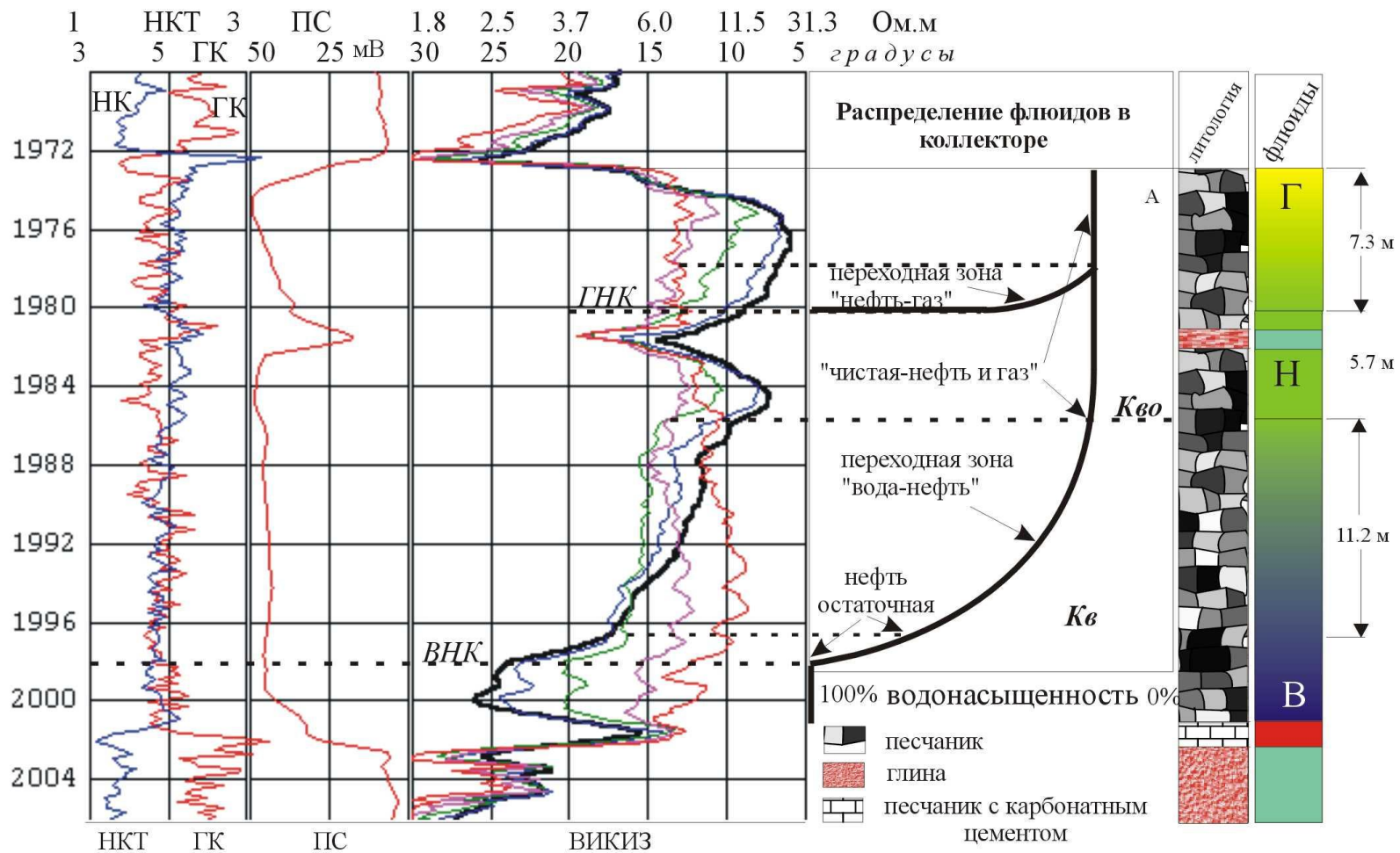
Рис.3. Разрез залежи пластов АС_7-8. Федоровское месторождение.
