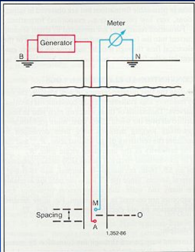
Схема измерений
