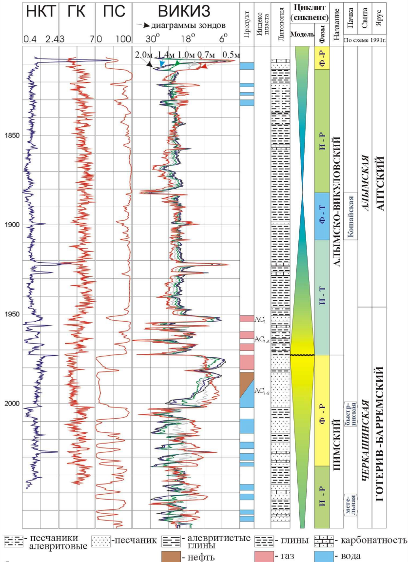
Рис. 2. Литостратиграфическая модель продуктивных готери-аптских отложений скважины 4614 Федоровского месторождения по данным ВИКИЗ.
