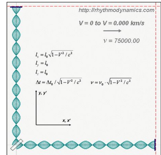
Фиг.3 Длины плеч, темп хода времени и частота зависят от скорости системы (по Лоренцу). Дополнительные стоячие волны в плечах не появляются, т.к. их длина, а значит и количество компенсируются зависимостью частоты источника волн от скорости системы в волновой среде.
