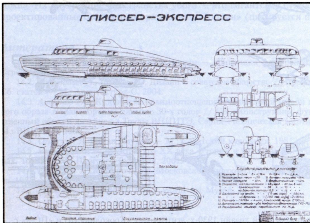
Владимир Мещерин. Глиссер-экспресс «ОСТА-25», 1936—1937
