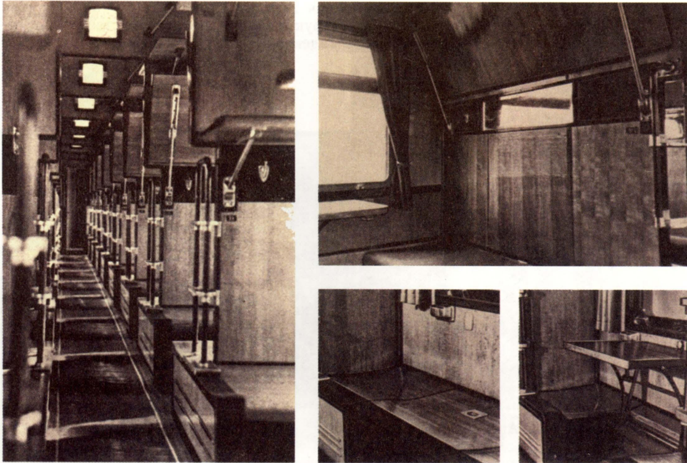
Ю. Соловьев, Ю. Сомов и др. Разработка цельнометаллического плацкартного вагона, 1946
