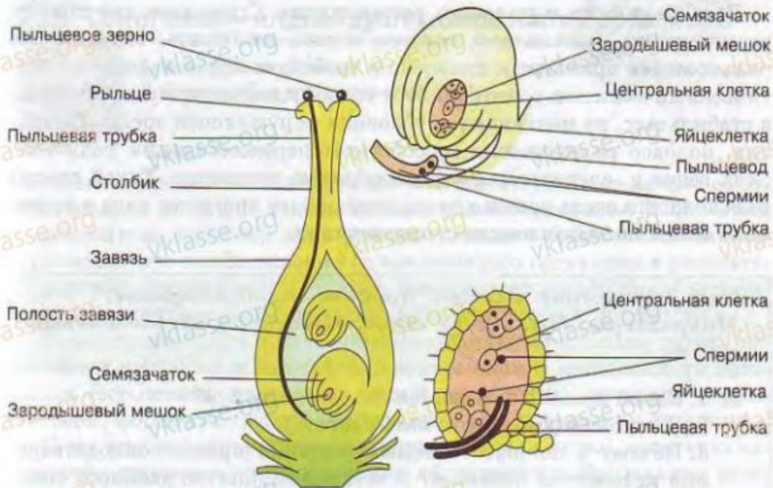
Рис. 53. Двойное оплодотворение у покрытосеменных
