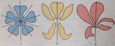
Рис. 75. Симметрия цветка:
