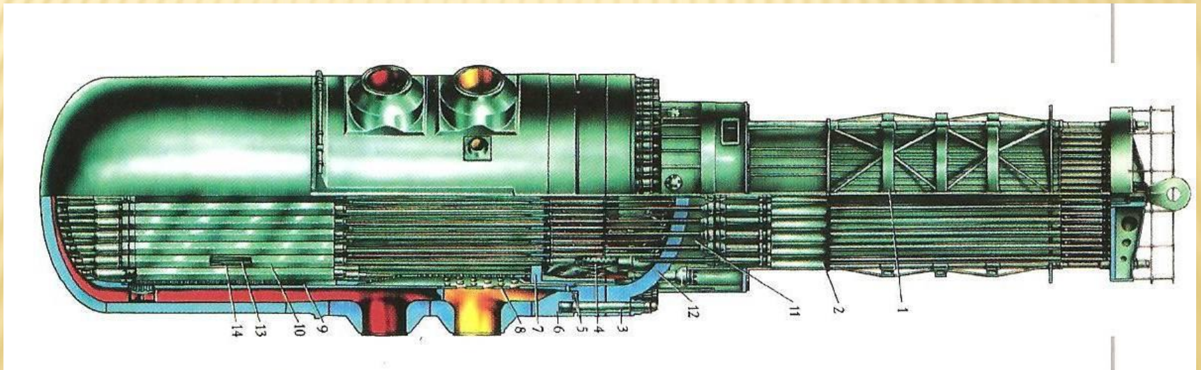
ВВЭР-1000
