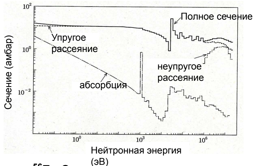
^{56}\text{Fe} Сечение (JENDL-3.3)
