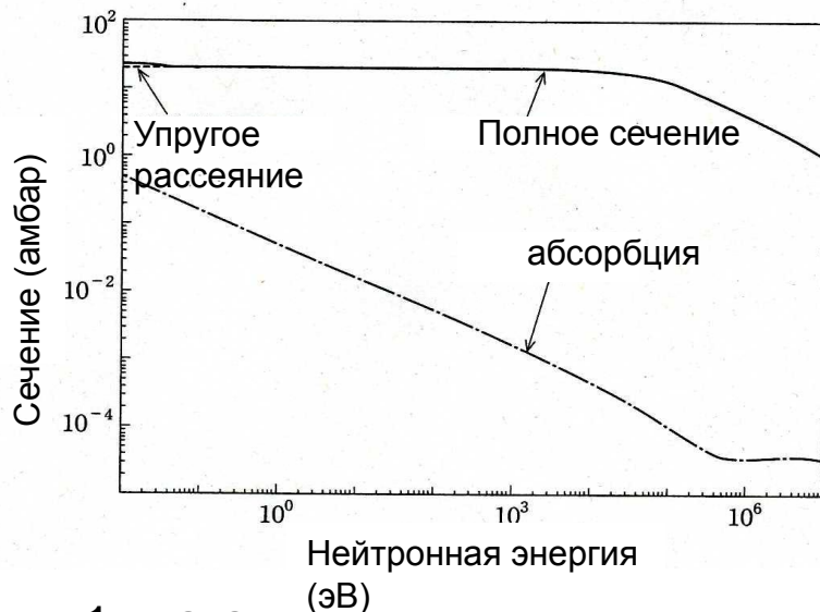
^{14}\text{C} Сечение (JENDL-3.3)
