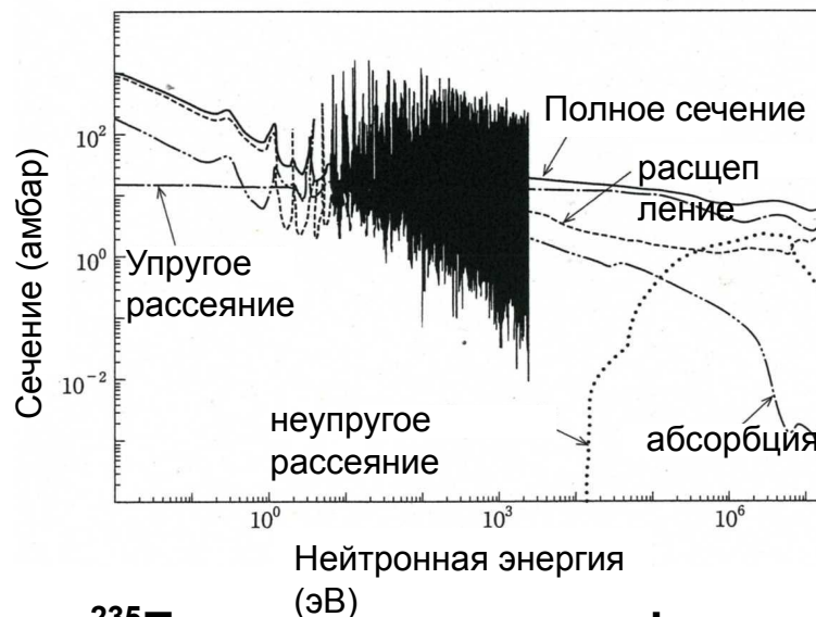
^{235}\text{U} Поперечное сечение \Sigma (JENDL-3.3)
