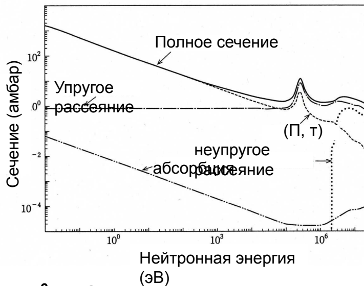
^6\text{Li} Сечение (JENDL-3.3)
