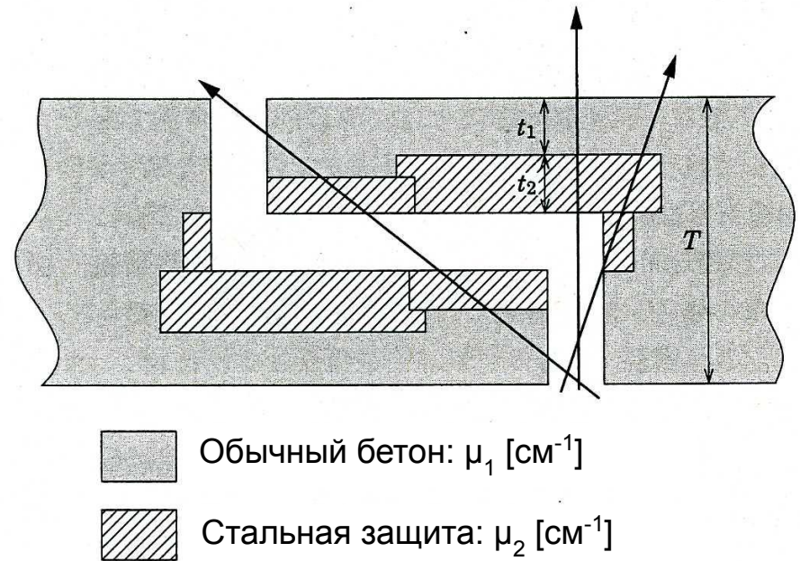
Рис. Компенсация экранирования для 2 изгибов канала
