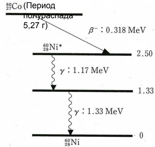
Рис. Распад схема ^{60}\text{Co}
