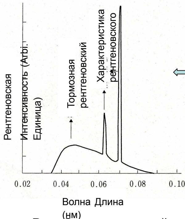
Рис. Энергетический спектр Рентгеновский из Mo
