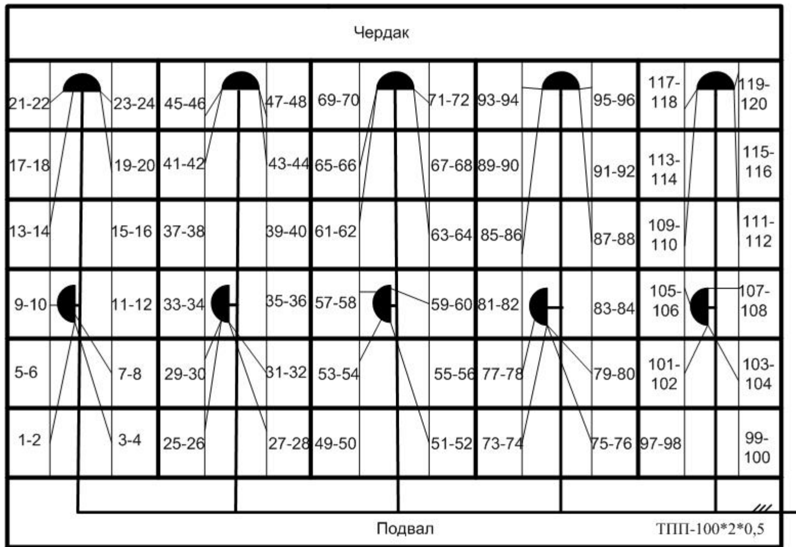
Рисунок 3 -Схема разводки кабеля внутри дома
