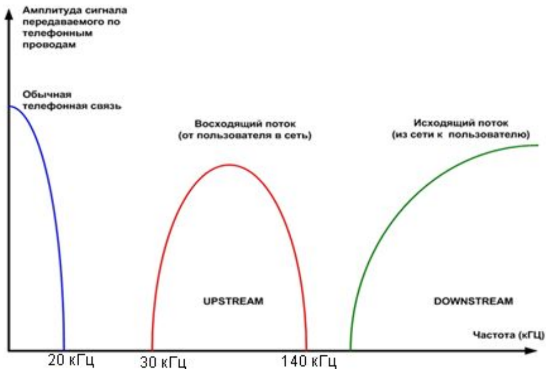
Рисунок 1 - Частотный диапазон для передачи сигналов телефонии и ADSL
