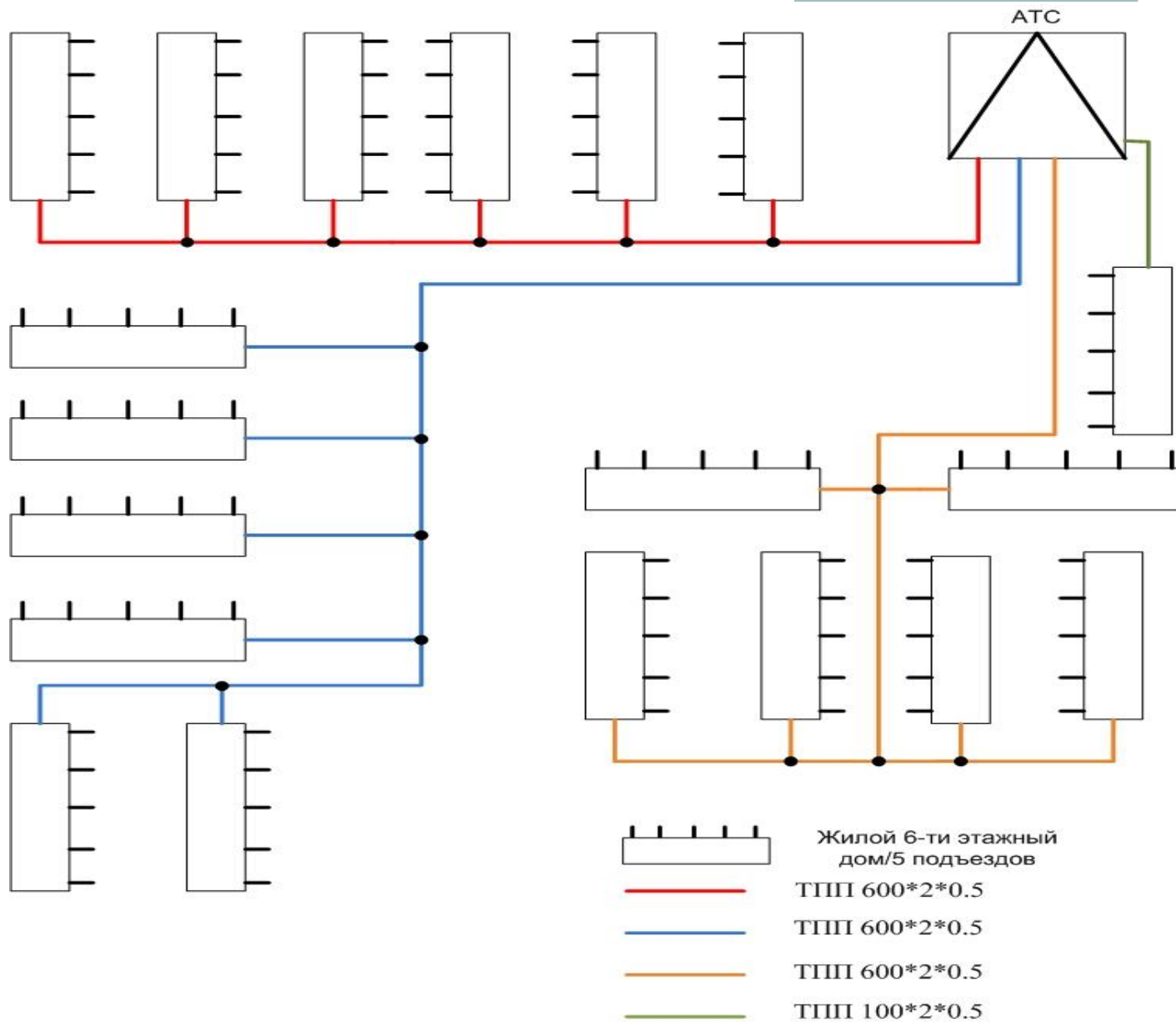
Рисунок 2 - Схема разводки кабеля по жилому массиву
