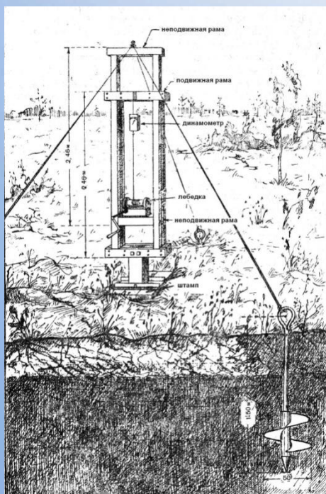
← Устройство (штамп) для передачи нагрузки на болото
