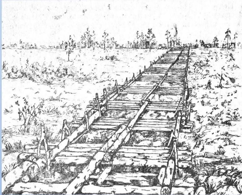
Вид опытного участка «пакетного» покрытия на болотном массиве с обжимными и продольными брусьями, выдерживающее 8-кратные проходы танка Т-34
