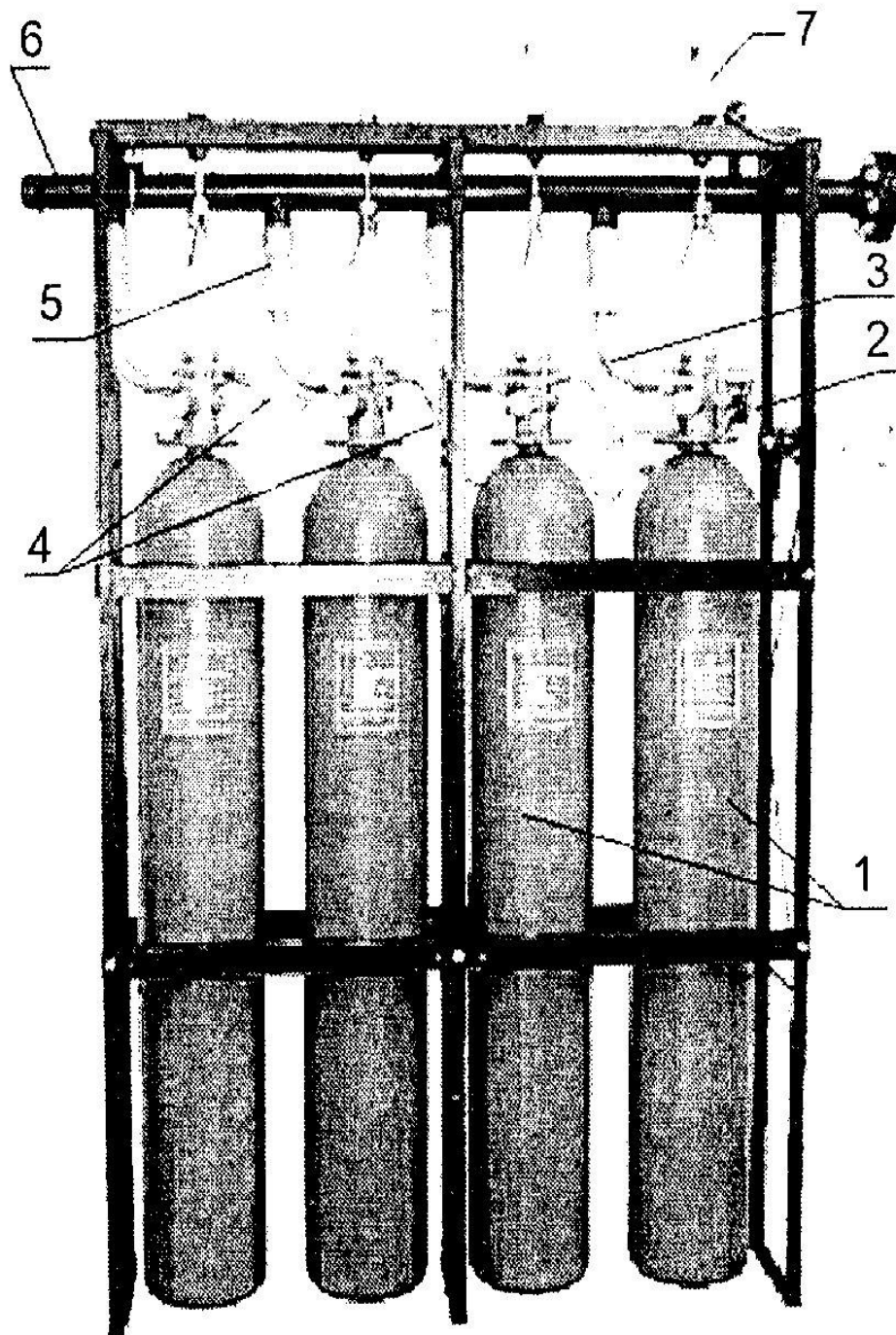
Рис. 3.4.4. Конструкция батареи с электромагнитным (ЗПУ ЭМК, первый модуль) и промежуточными пневмоклапанами модулей: 1 — модули МГП; 2 — ЗПУ; 3 — рукав высокого давления (РВД); 4 — РВД пневмопуска; 5 — обратный клапан; 6 — общий коллектор; 7 — направления тушения
