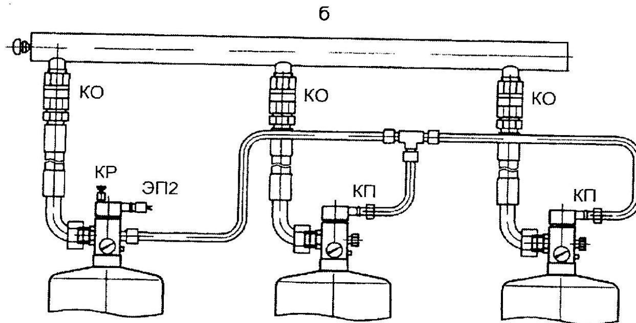
Рис. 3.4.5. Схема электропневматического пуска батареи УАГП: а — последовательный пуск; б — параллельный пуск
