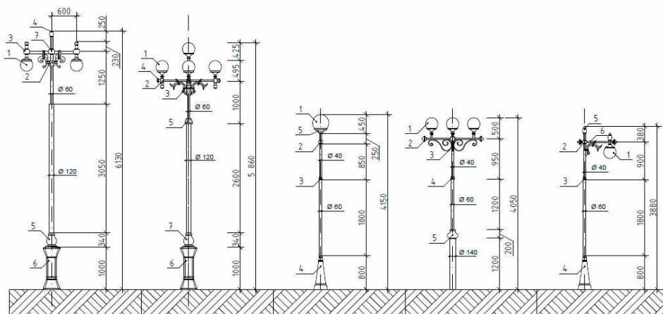
Фонарь ФБ-2
