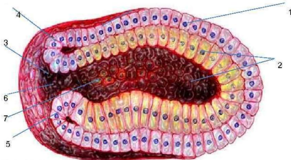
Рис. Гаструла ланцетника.
