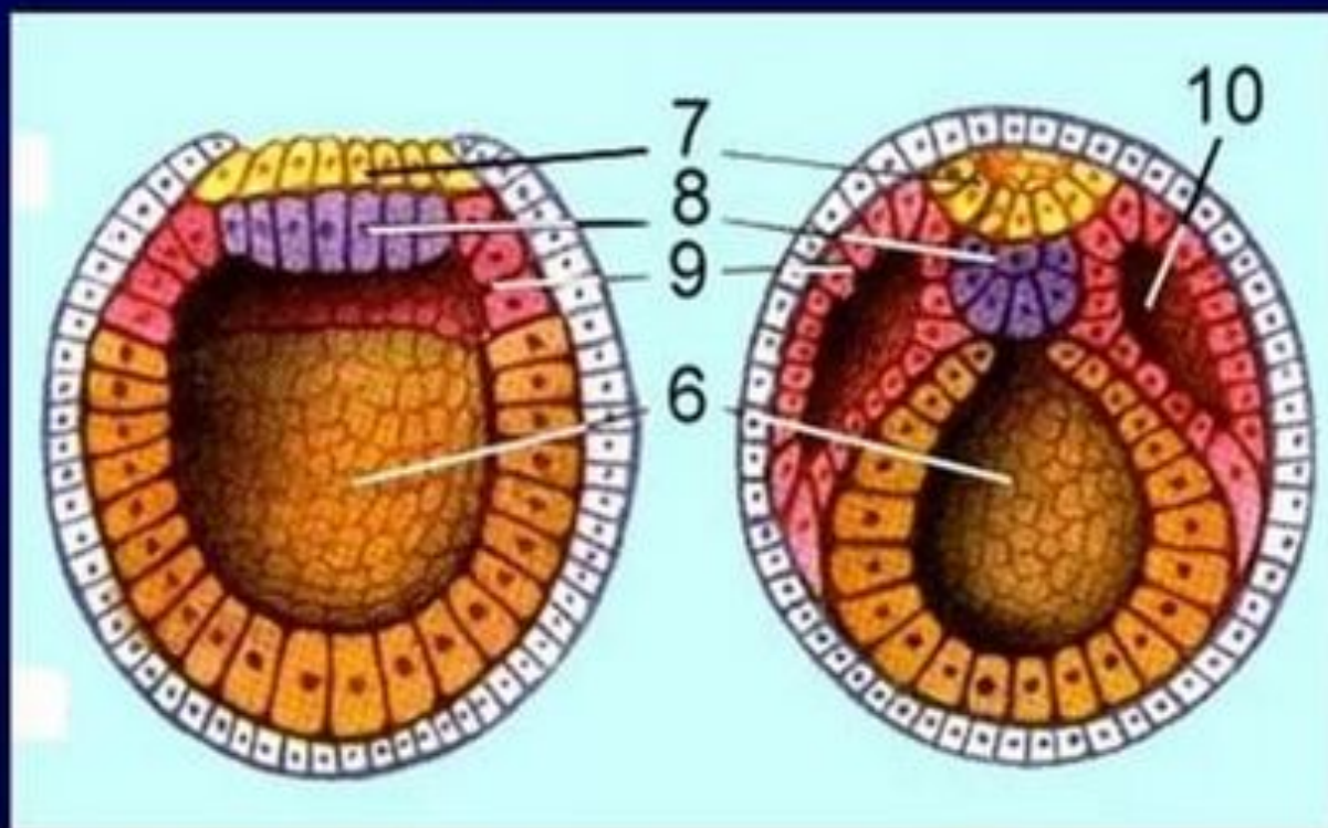
Ранняя нейрула
