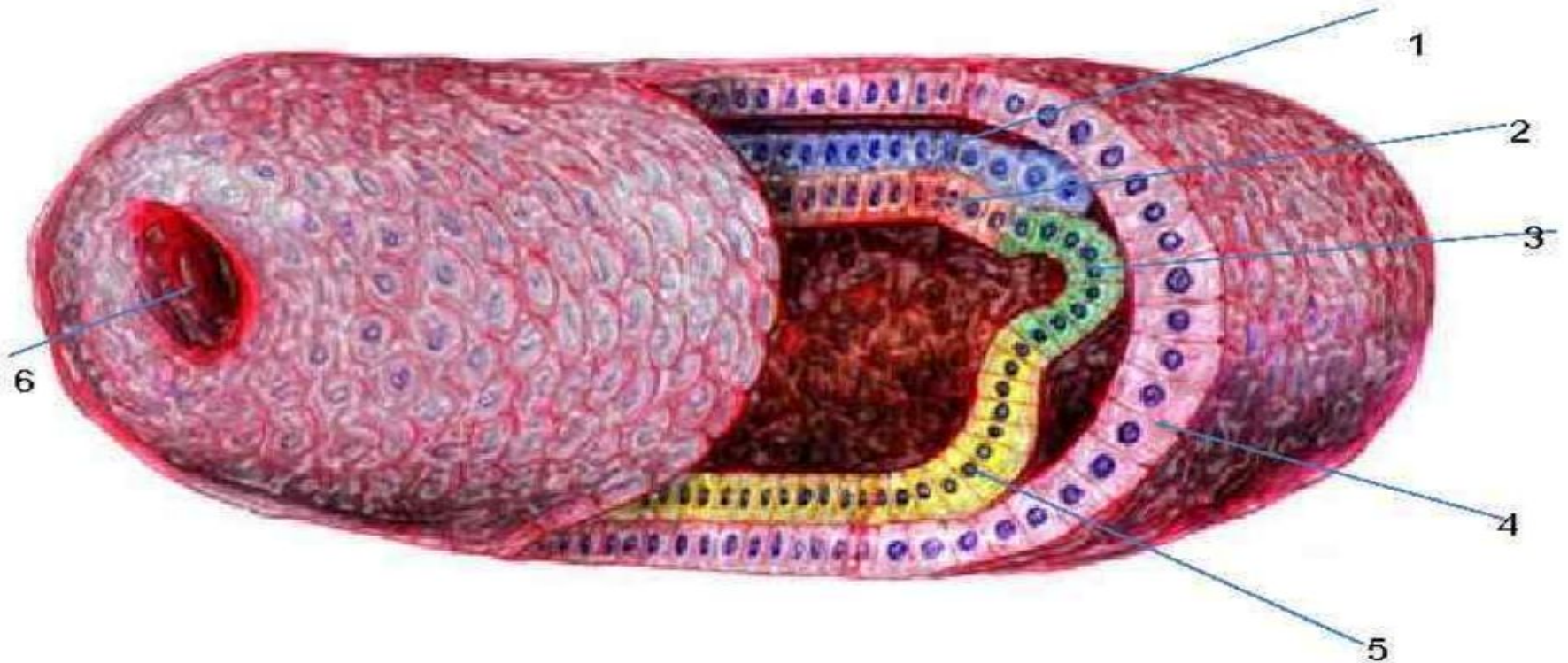
Рис. Формирование осевых закладок органов: 1 – нервная пластинка; 2 – хорда; 3 – мезодерма; 4 – эктодерма; 5 – энтодерма; 6 – первичное ротовое отверстие.
