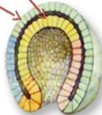
Гастрюла
