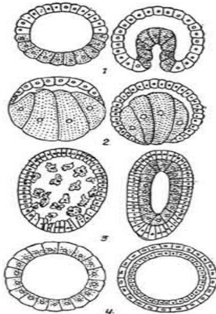
Рис. 46. Способы гастрюляции:
