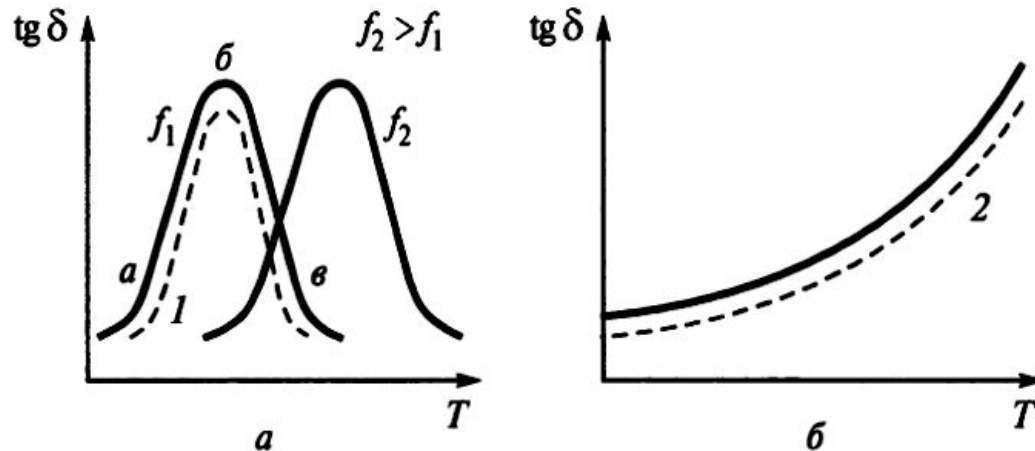
Рис. 4.5. Схематическое изображение температурной зависимости тангенса угла диэлектрических потерь \text{tg } \delta , обусловленных дипольно-релаксационной (а) и ионно-релаксационной (б) поляризациями: образующие \text{tg } \delta , вызванные: 1 — дипольно-релаксационной поляризацией; 2 — ионно-релаксационной поляризацией
