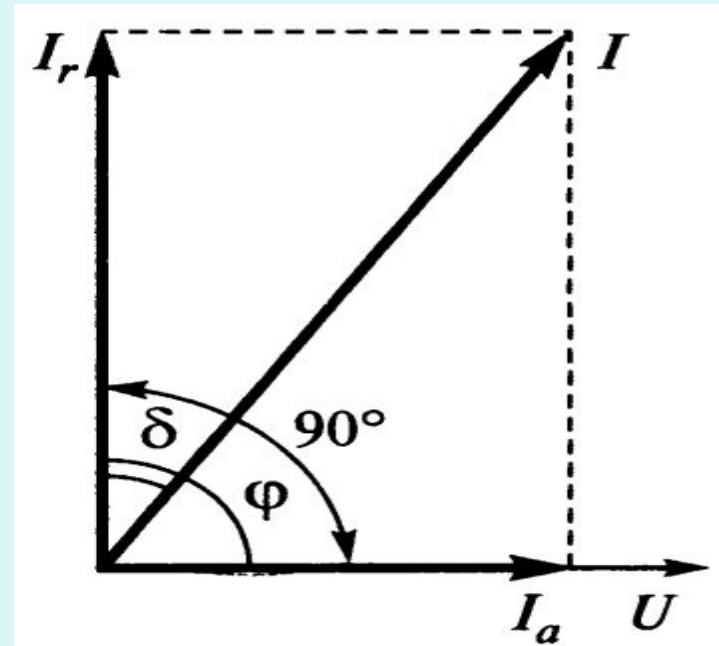
Рис. 4.1. Векторная диаграмма диэлектрика с потерями
