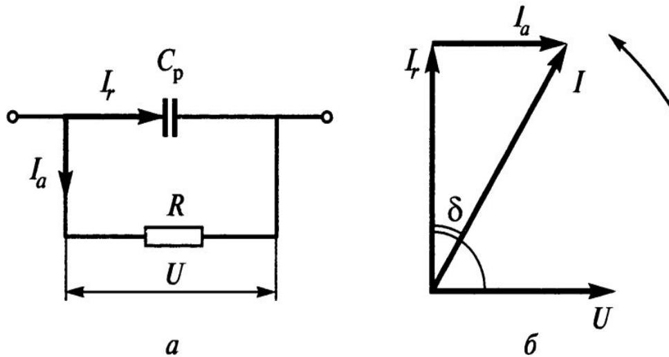
Рис. 4.2. Параллельная эквивалентная схема замещения диэлектрика с потерями (а) и векторная диаграмма токов в ней (б)
