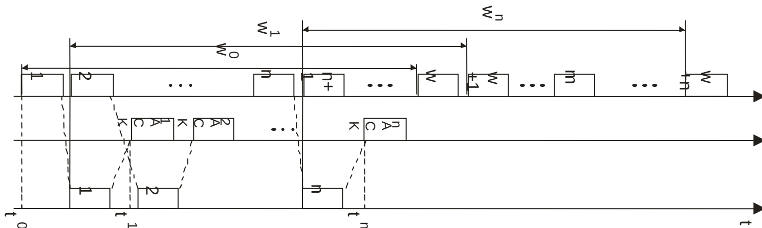
Скользящее окно - квитанции
