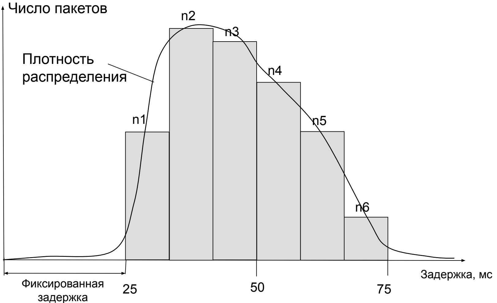
Гистограмма распределения задержек
