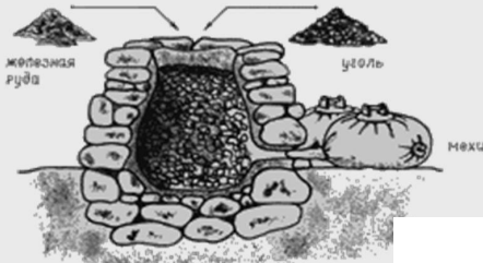
Получение губчатого железа в каменном горне
