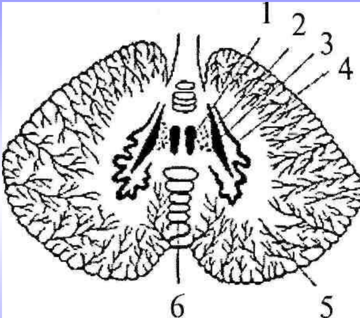
Ядра мозжечка: 1 — ядро шатра; 2 — шаровидное ядро; 3 — пробковидное ядро; 4 — зубчатое ядро; 5 — полушария мозжечка; 6 — червь мозжечка
