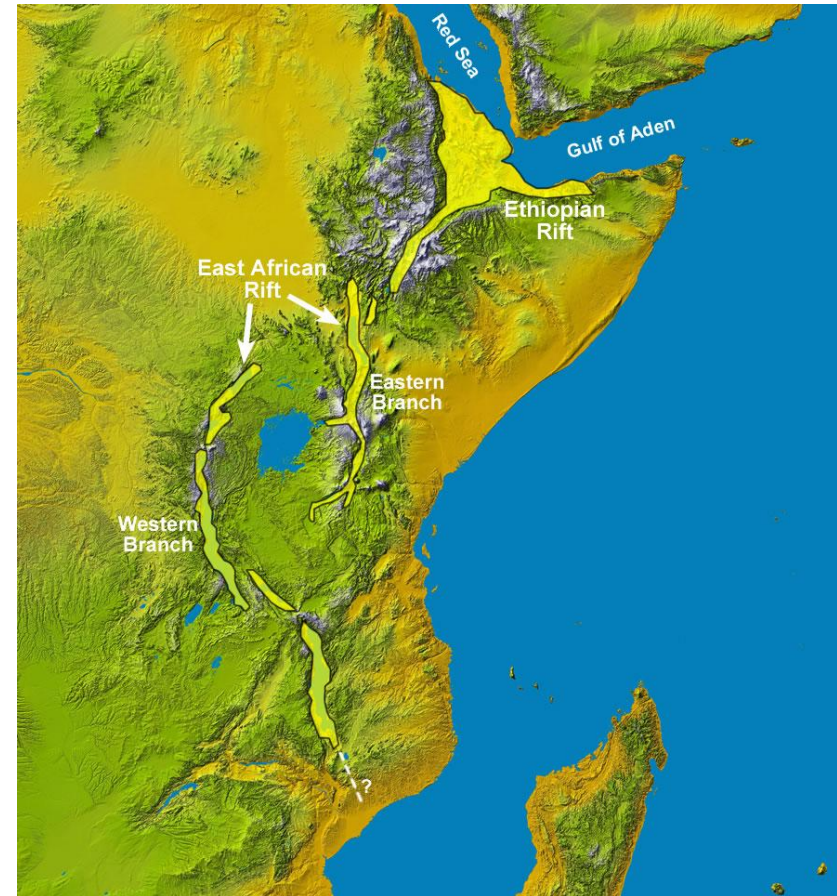
Восточно-Африканская рифтовая система
