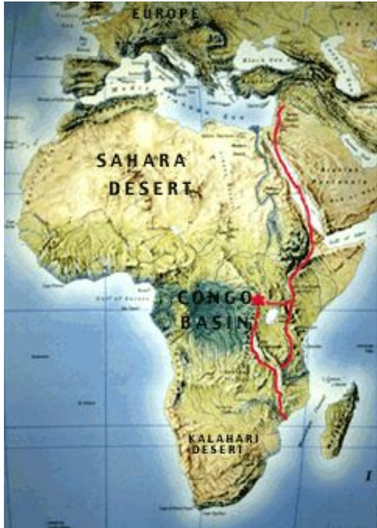
Общая схема тектонических разломов
