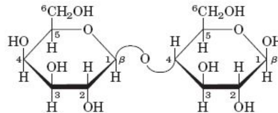
Lactose ( \beta form)
