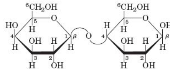
Lactose ( \beta form)
