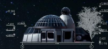
Фасад в осях Е-Н M1:200
