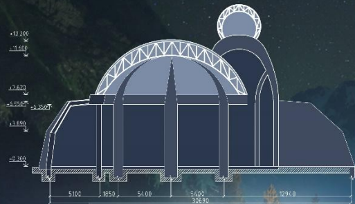
Разрез А-А M1:100
