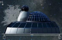
Фасад в осях Н-О M1:200
