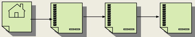
Линейная структура
