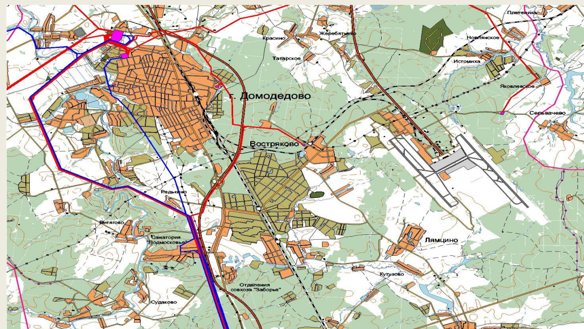
Векторные данные
