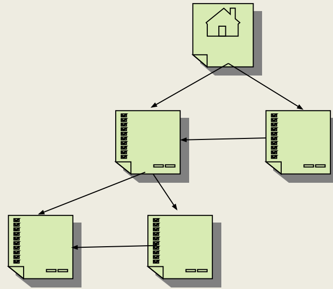
Структура «паутина»
