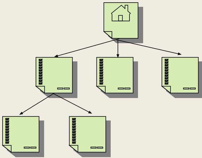
Структура «дерево»
