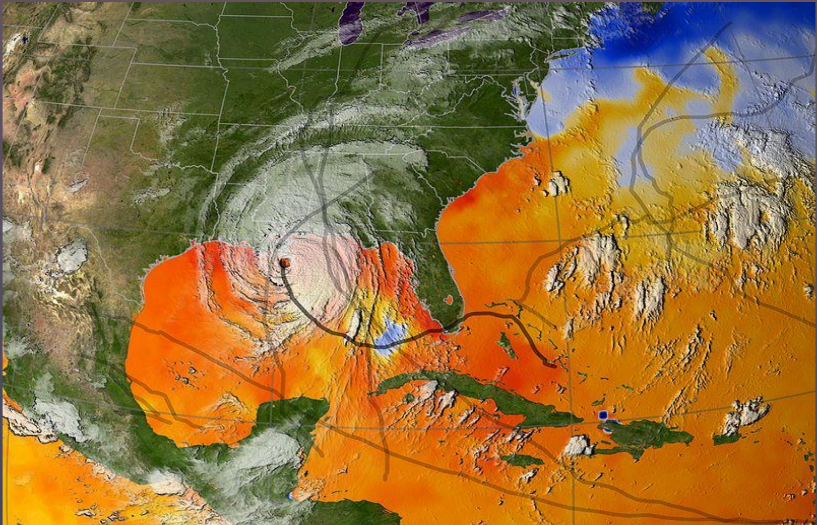
Траектория урагана Катрина на фоне облачности и температуры поверхности моря на 29 августа 2005 года.
