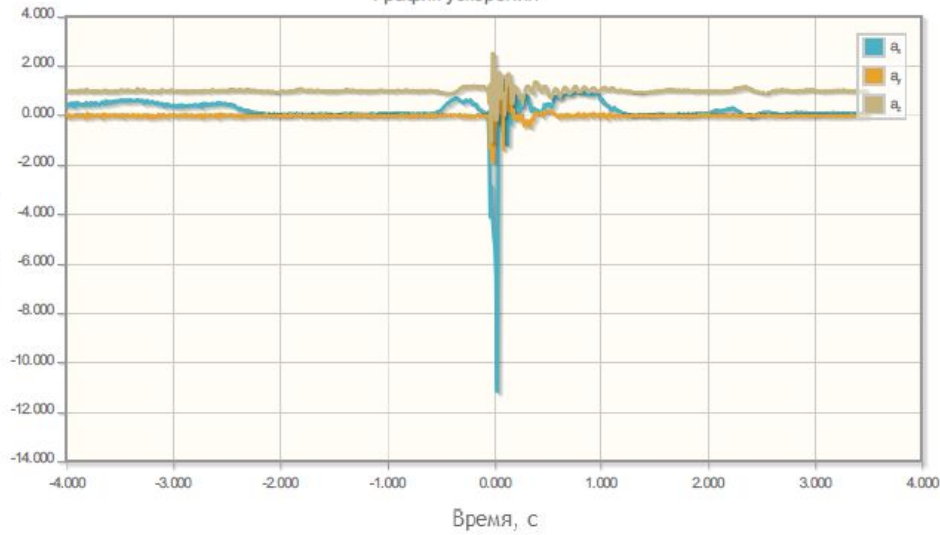
График ускорения
