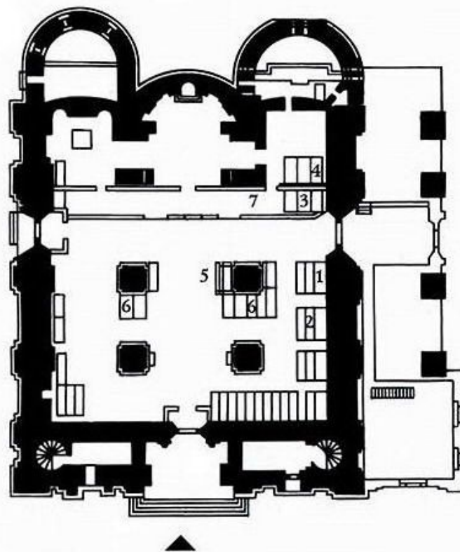
Кремль Московский. Архангельский собор (план).
