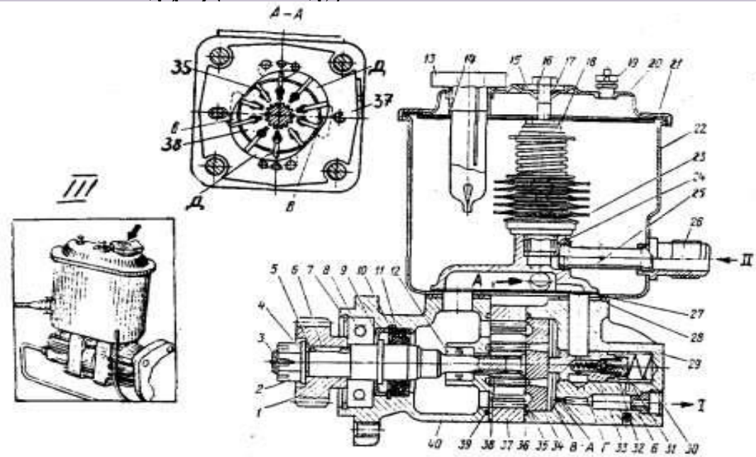
Рис. 3.7. Насос рулевого гидроусилителя автомобилей КамАЗ-4310, КамАЗ-5320:
