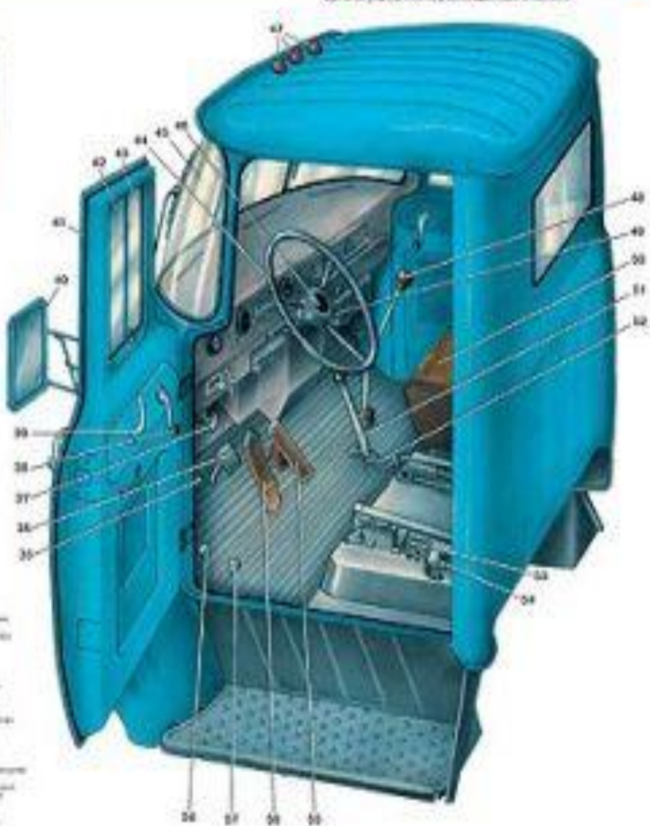
Органы управления, расположенные в кабине
