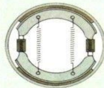
барабанный тормоз отключен
