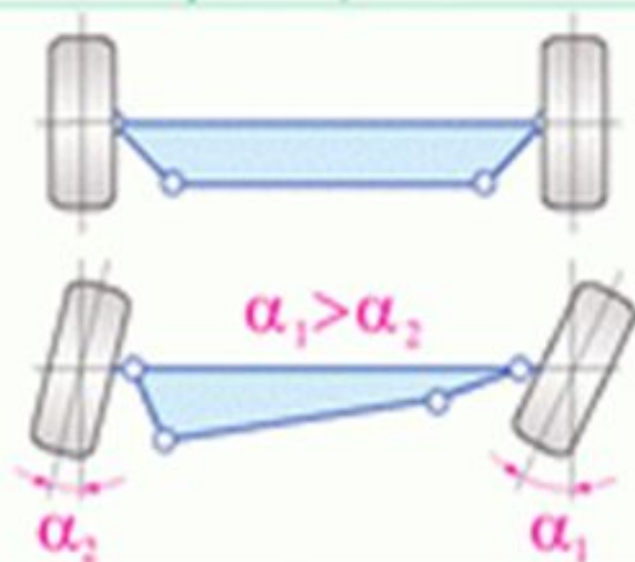
Рулевая трапеция
