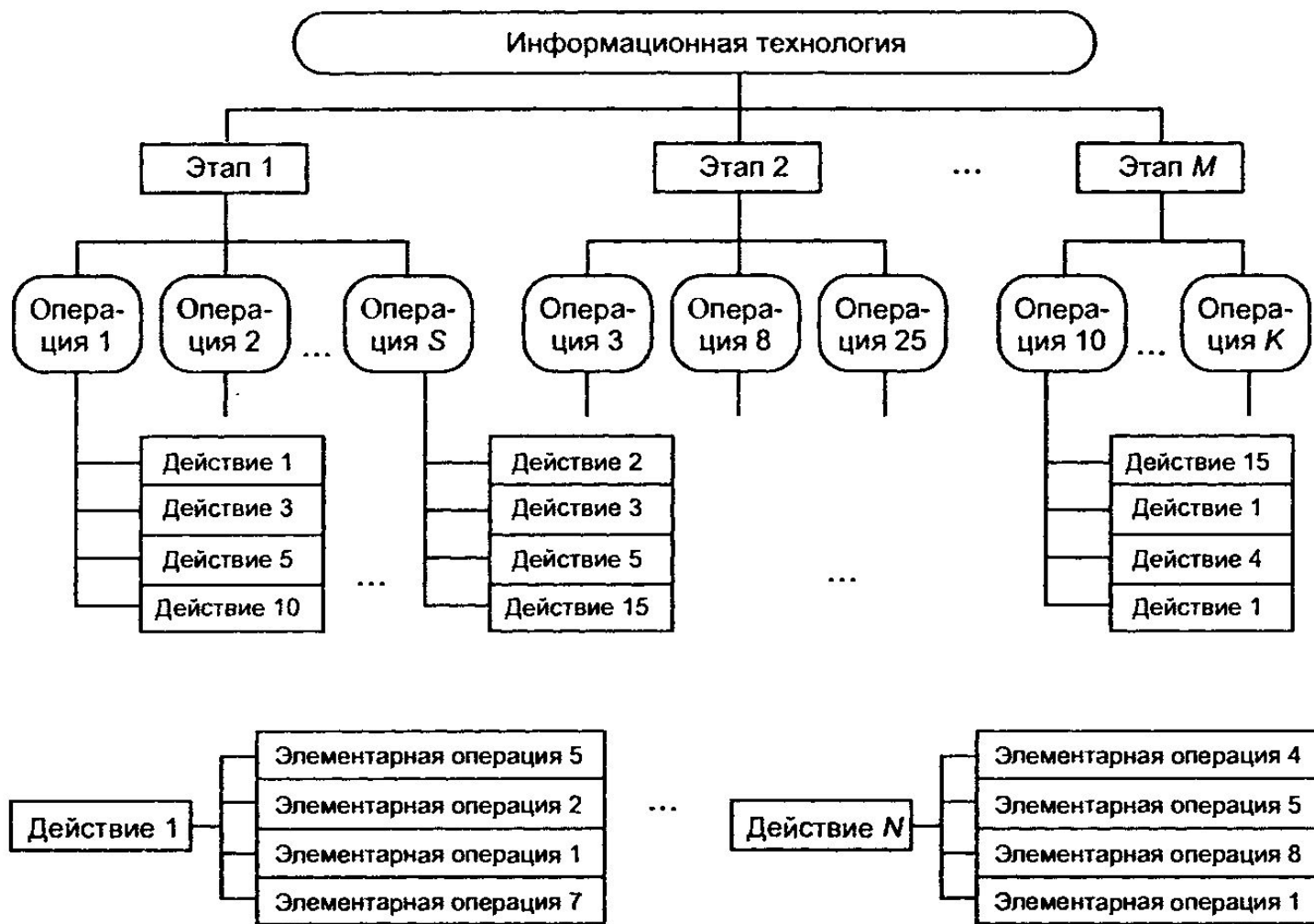
Рис. 5.3. Представление информационной технологии в виде иерархической структуры, состоящей из этапов, действий, операций
