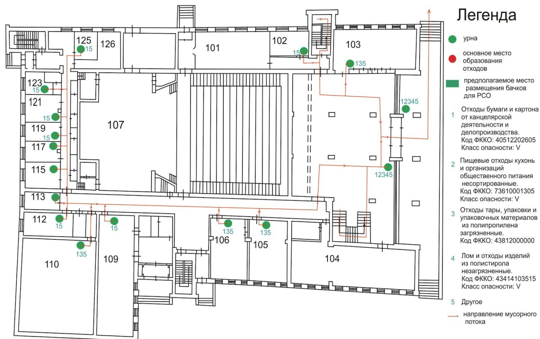
I этаж Территориальная схема по обращению с отходами 5-го корпуса ЧелГУ
