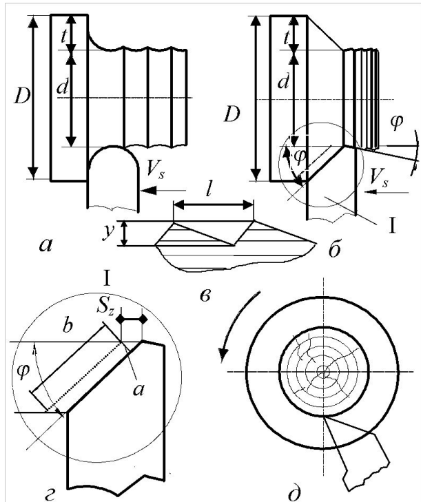
Рис. 84. Радиальное точение: a – черновое; б, д – чистовое; в – шероховатость поверхности; г – поперечные размеры среза
