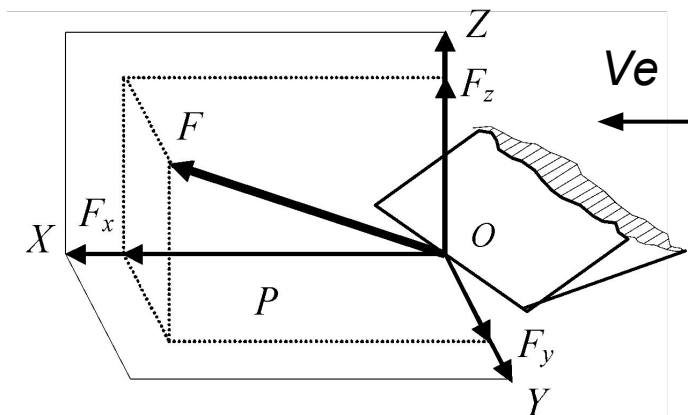
Рис. 28. Составляющие силы резания
