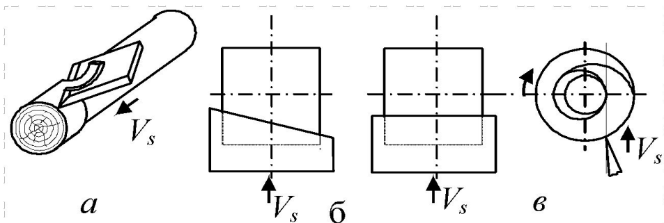
Рис. 65. Тангентальное точение: a – с продольной подачей; б, в – с поперечной подачей
