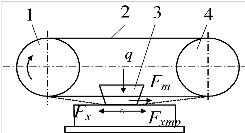
Рис. 88. Схема шлифования древесины
