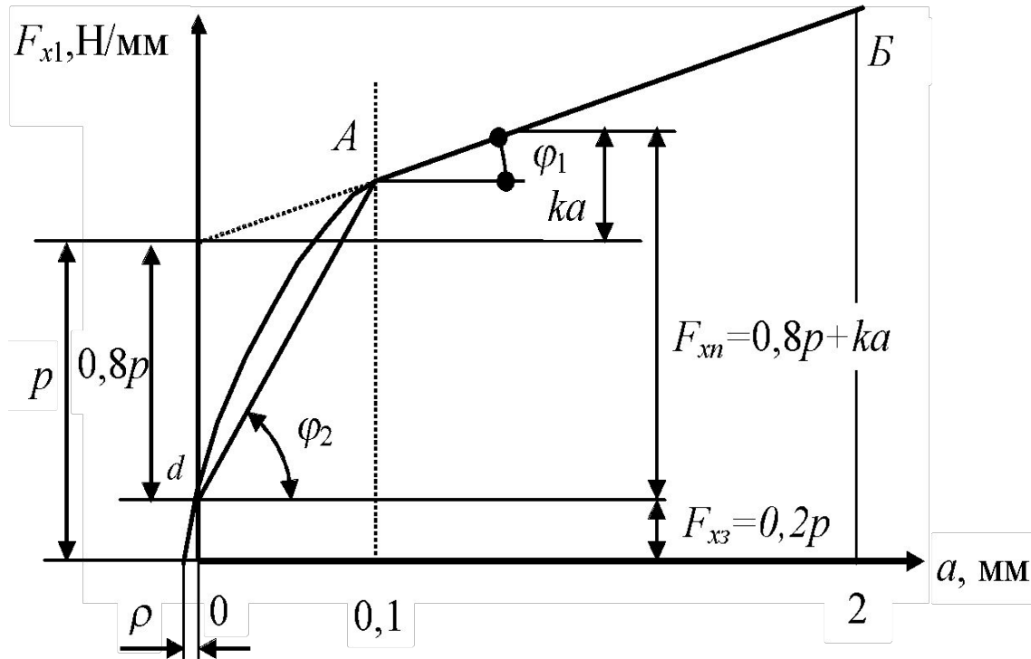
Рис. 32. Зависимость касательной силы от толщины срезаемого слоя
