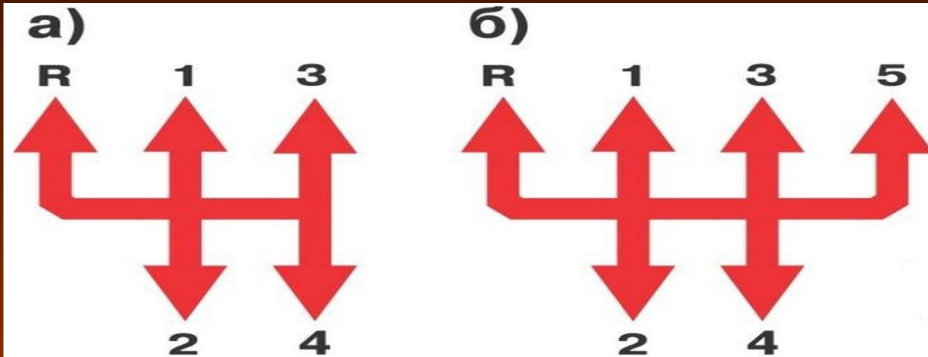
Рис. 3. Схема переключения передач: а - для четырехступенчатой коробки передач; б - для пятиступенчатой коробки
