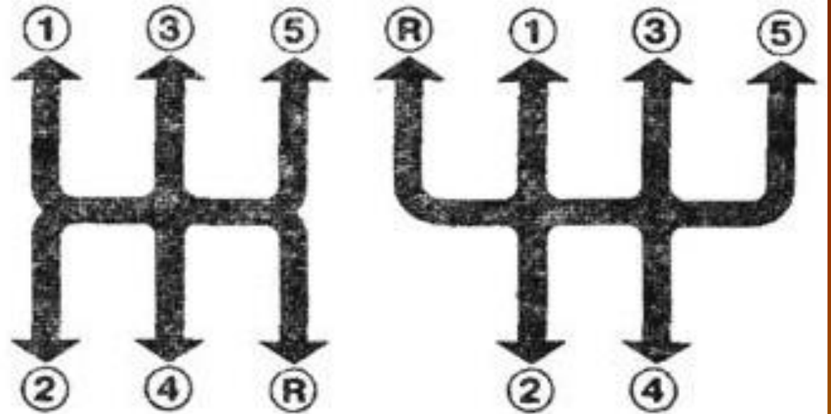
5-ти ступенчатая коробка передач
