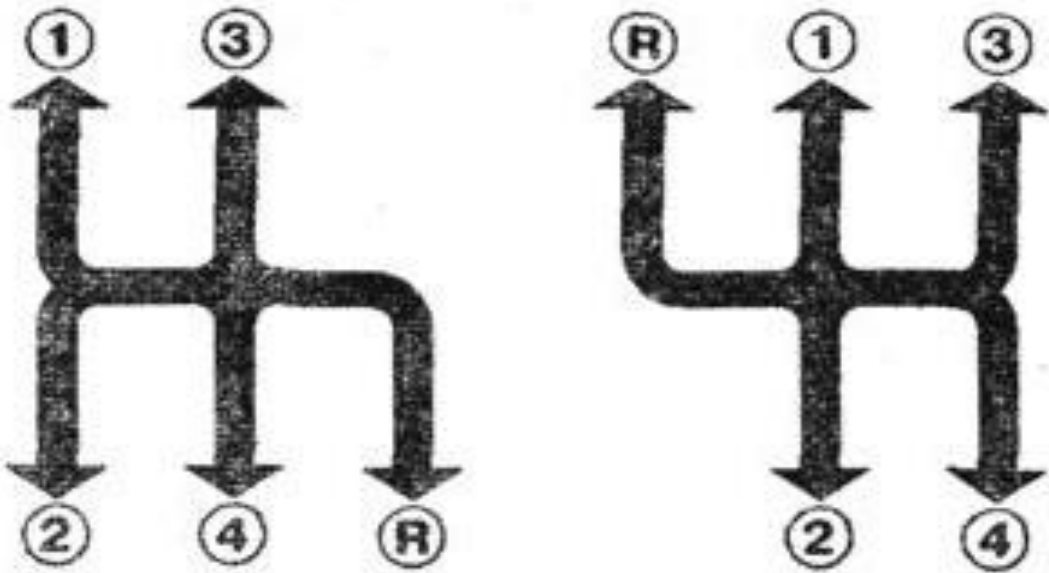
4-х ступенчатая коробка передач
