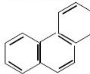
Фенантрен
