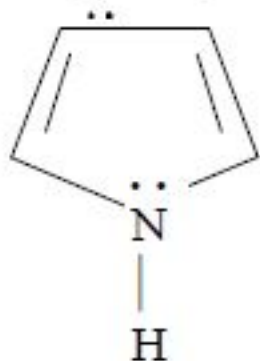
пиррол
