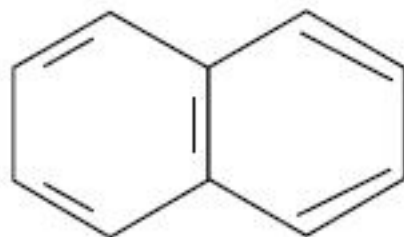
нафталин
