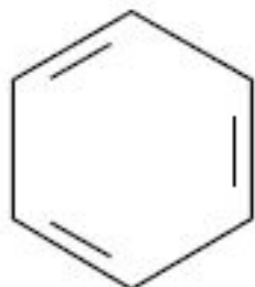
бензол
