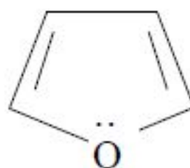
фуран
