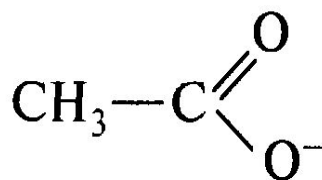
ацетат-ион
