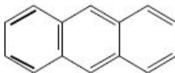
Антрацен
