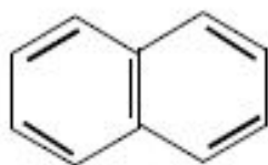
Нафталин
