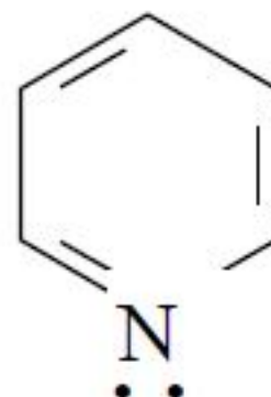
пиридин
