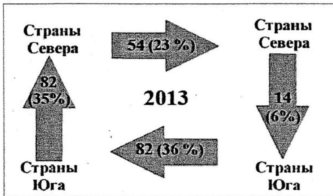
Рис. 1 – Глобальное распределение мигрантов по регионам прибытия и выбытия в 2013 г., млн. чел.
