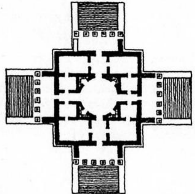
А. Палладио. Вилла Ротонда. Фасад и план. Италия. XVI в.
