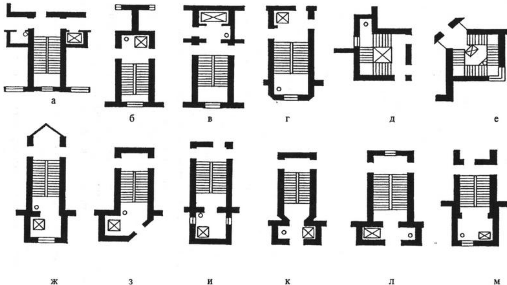
Рис. 2.17. Типы лестнично-лифтовых узлов, используемых при реконструкции жилых домов: а...в - лифты и мусоропроводы выполнены в помещениях, примыкающих к лестничным клеткам; г...е - лифты и мусоропроводы вписаны в габариты лестничной клетки; ж...м - объемы пристроек к торцу лестничной клетки (для зданий, которые ориентированы на дворовой фасад и имеют ограниченные габариты)
