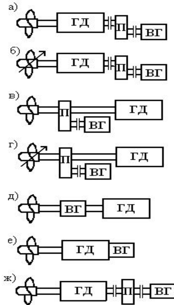
Варианты компоновки валогенераторов П — зубчатая передача; а, б — П и ВГ с ВФШ и ВРШ соответственно; в, г — П на промежуточном валу и ВГ с ВФШ и ВРШ соответственно; д — ВГ установлен на промежуточном валу; е — ВГ установлен на носовом торце ГД; ж — планетарная передача с переменным передаточным числом, установленная на носовом торце ГД
