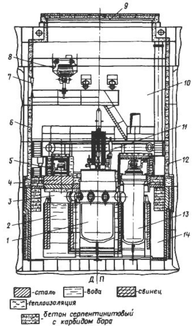
Размещение АППУ в защитной оболочке лихтеровоза-контейнеровоза «Севморпуть»
