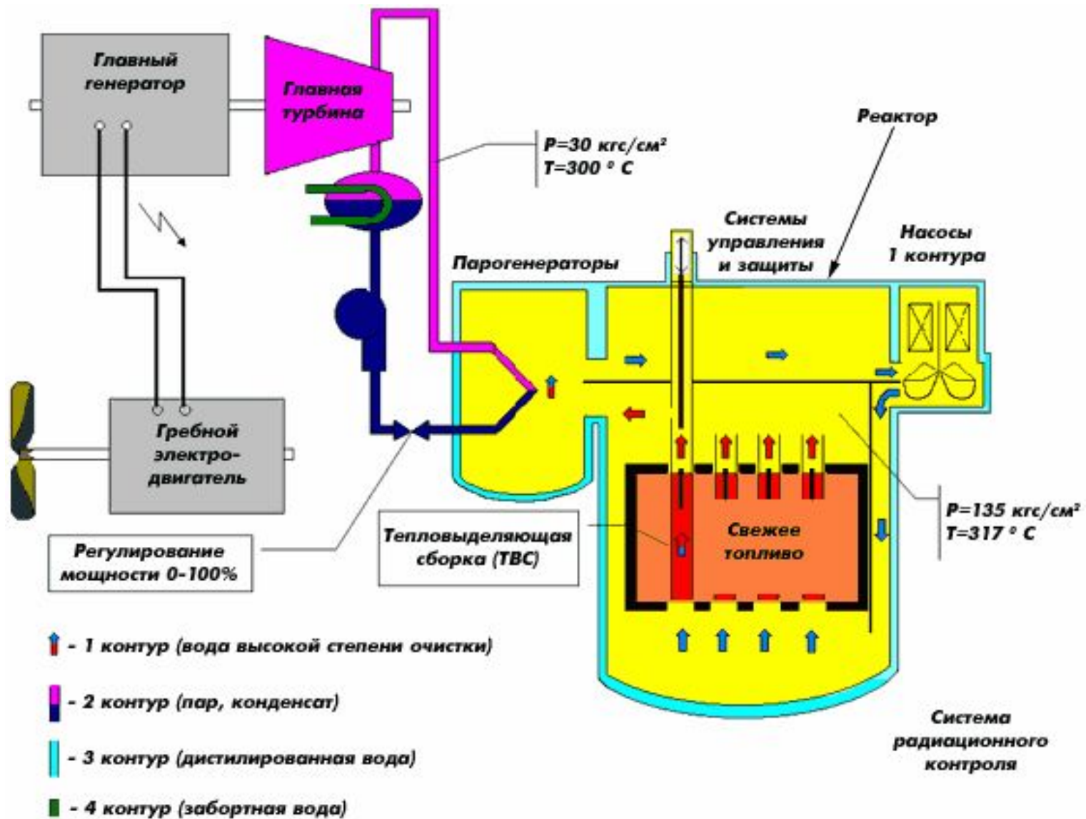
Принцип действия АППУ
