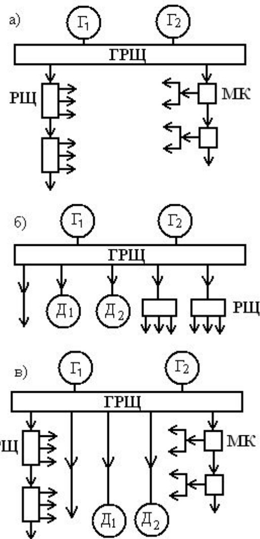
Различные системы распределения электроэнергии а — магистральная; б — фидерная (радиальная); в — смешанная
