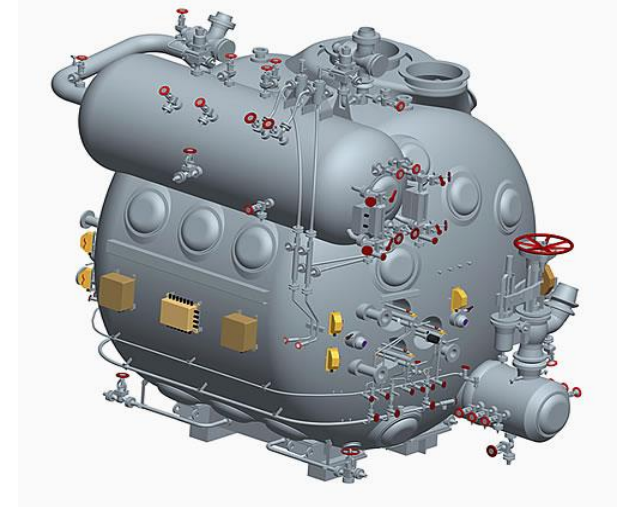
Схема и внешний вид главного котла типа КВГ-6М
