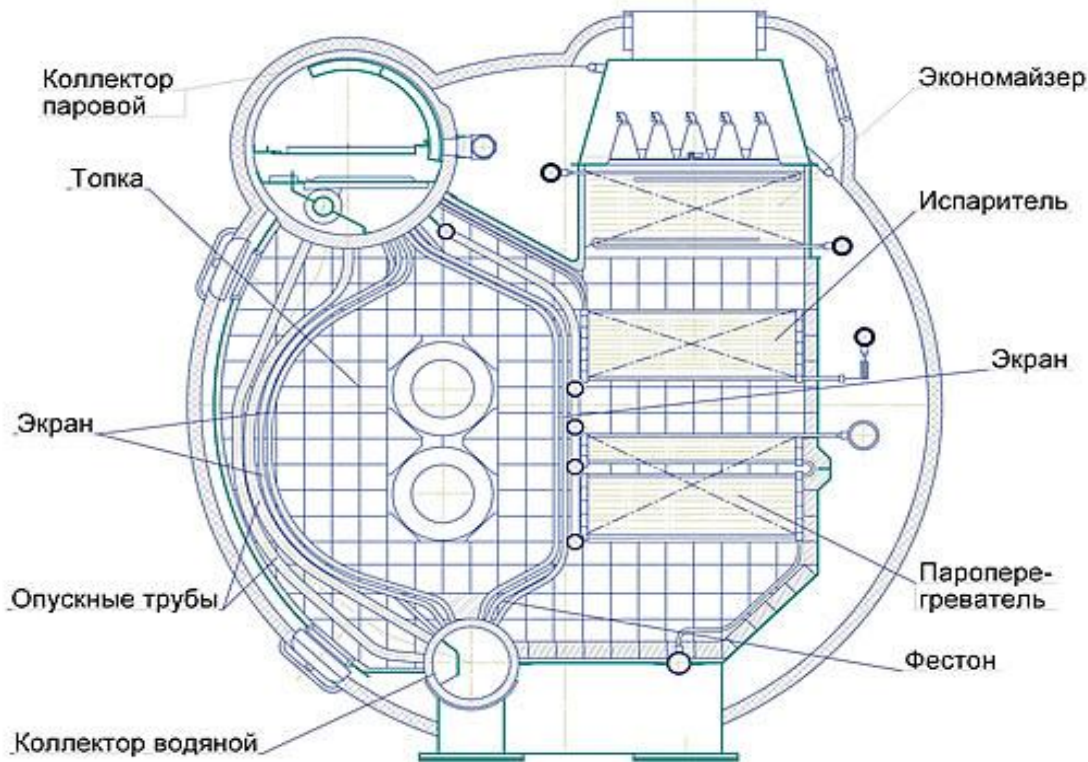
Схема и внешний вид главного котла типа КВГ-6М
