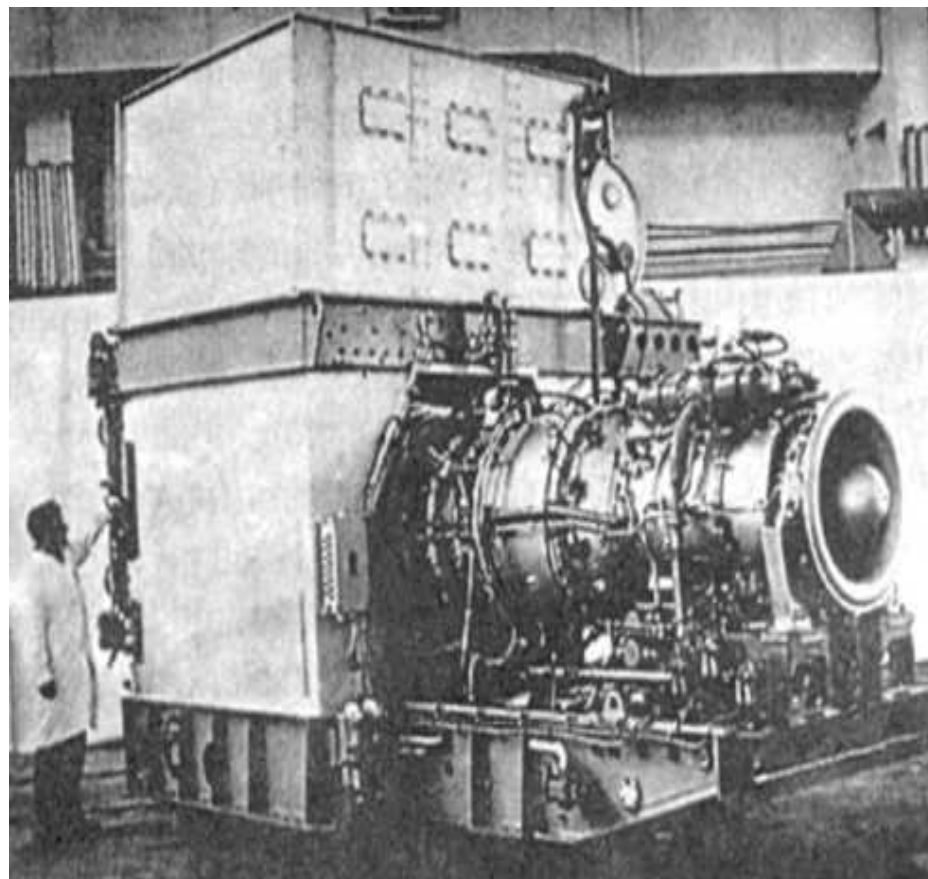
Главный газотурбинный агрегат с теплоутилизационным контуром пр. 1164
