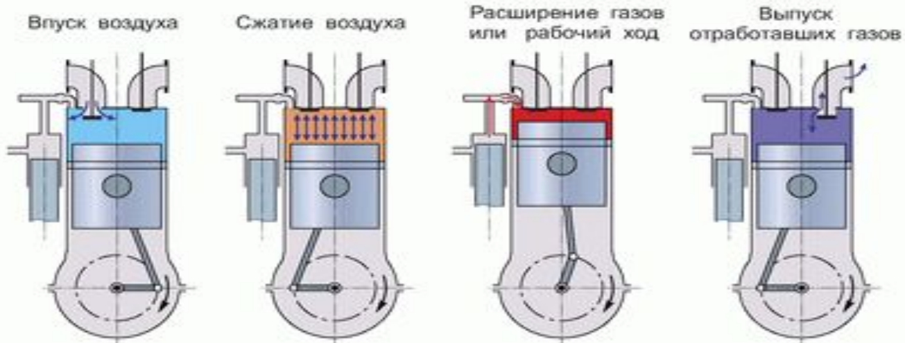
Принципы работы ДВС Схема работы четырехтактного дизеля
