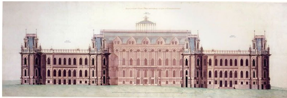
Первоначальный (неосуществленный) проект фасада Большого дворца. Чертеж нач. XIXв. (с оригинала М.Ф. Казакова конца 1780-х гг.). Музей архитектуры им. А.В. Щусева.
