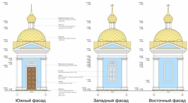
Южный фасад
