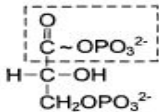
1,3-Бисфосфоглицерат
