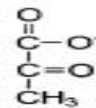
Пируват
