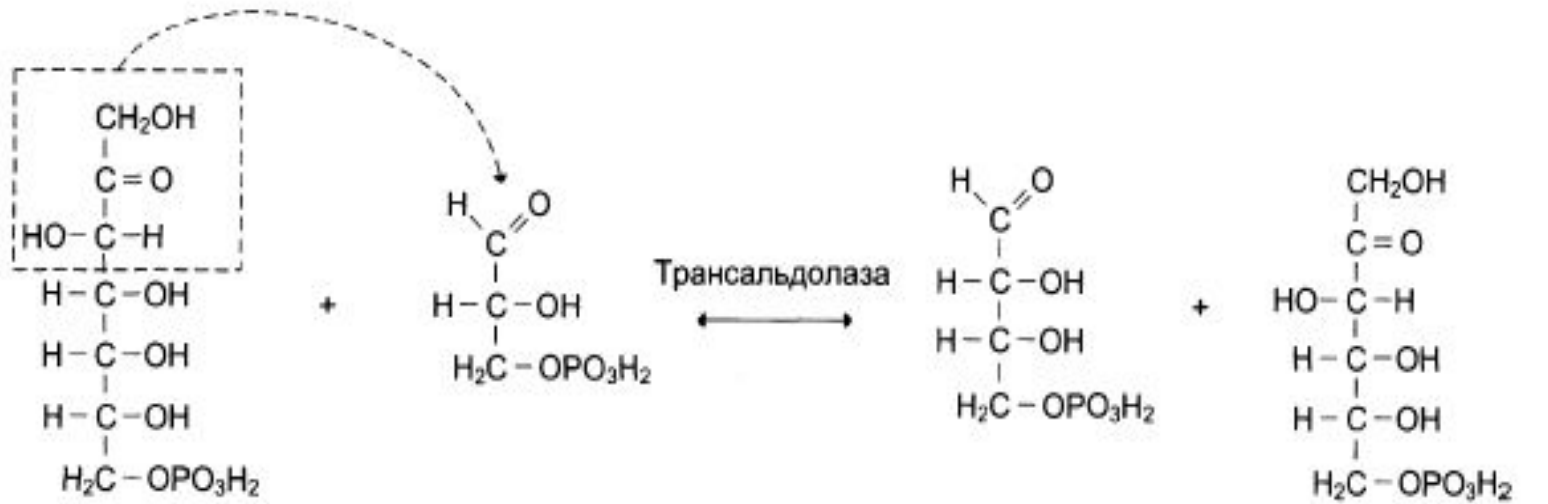
Седогеулозо-7-фосфат
