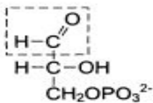
Глицеральдегид-3-фосфат
