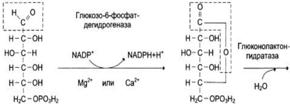
Глюкозо-6-фосфат
