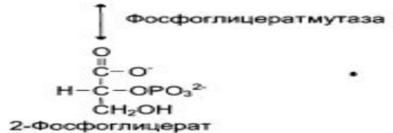
2-Фосфоглицерат
