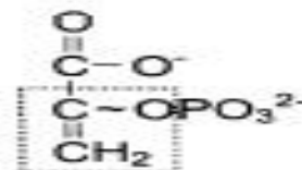
Фосфоенолпируват
