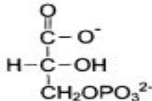
3-Фосфоглицерат
