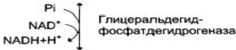
Глицеральдегид-3-фосфат
