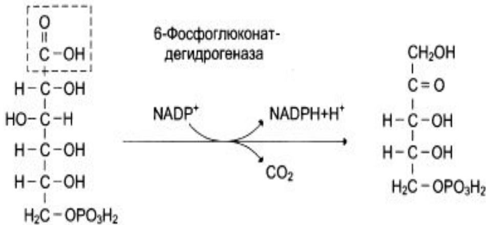
6-Фосфоглюконат
