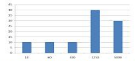
Гистограмма размеров ледяных полей D , м (январь)
