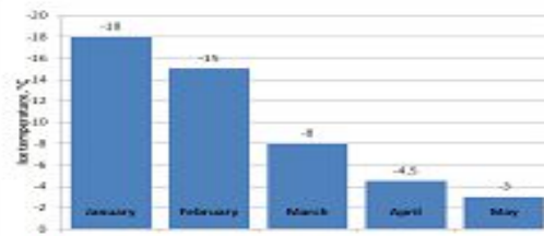
Гистограмма температуры льда T_i , °C
