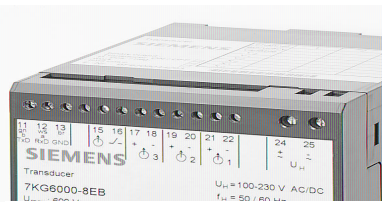
SIMEAS T
