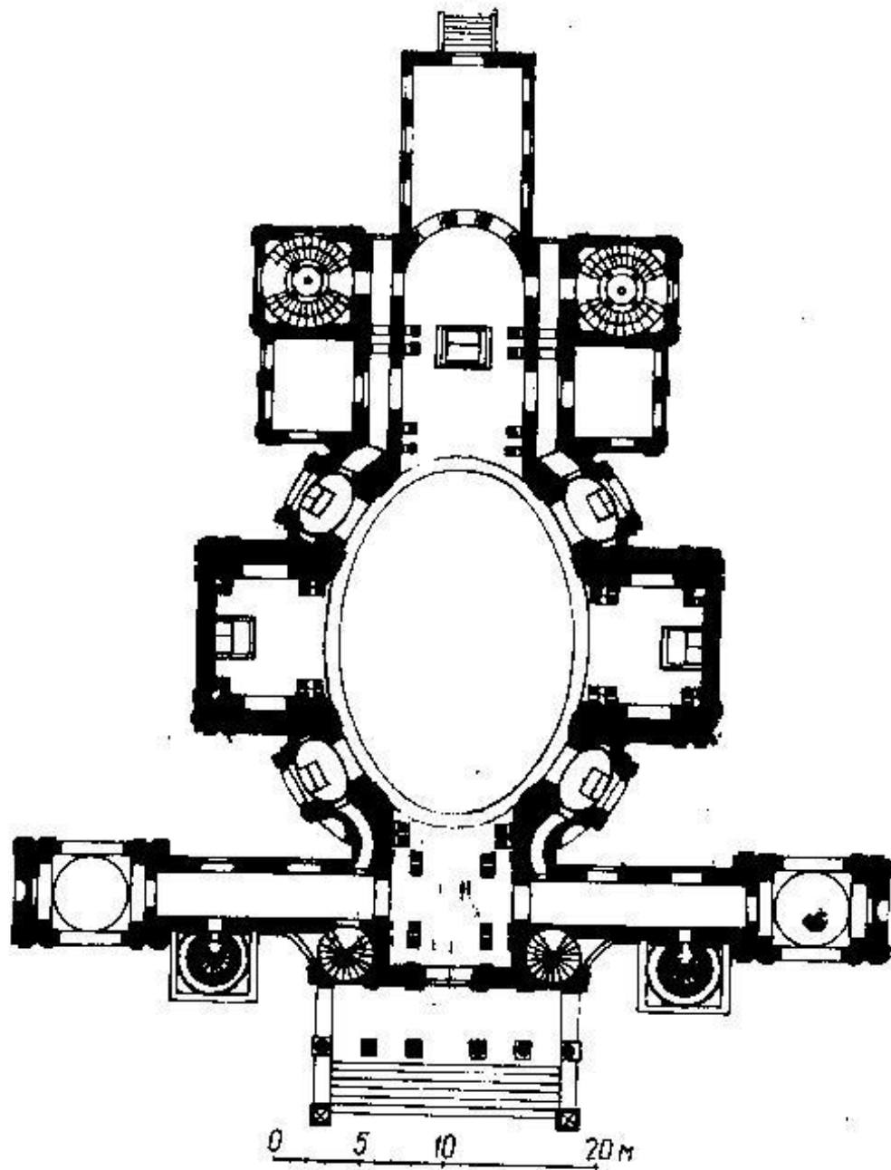
113. Церковь Карла Борромея в Вене, 1716-1737 гг. Арх. И.-Б. Фишер фон Эрлах. План
