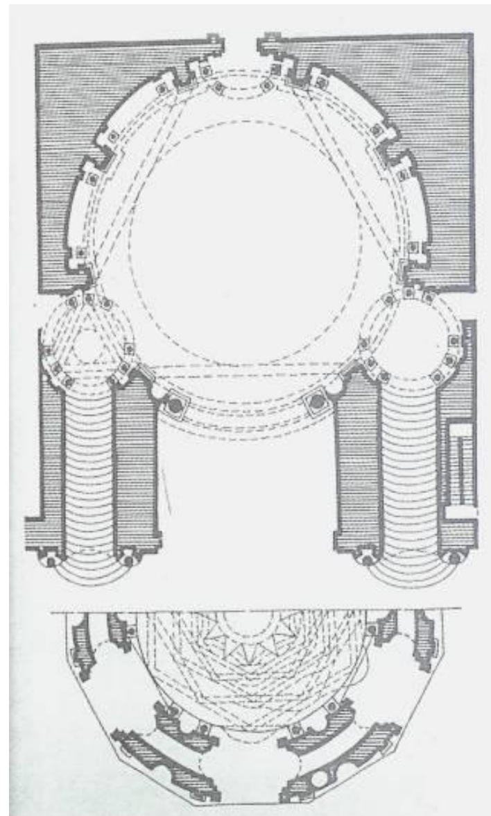
Капелла Сан – Синдоне в Турине. 1668 г. Арх. Гварино Гварини.
