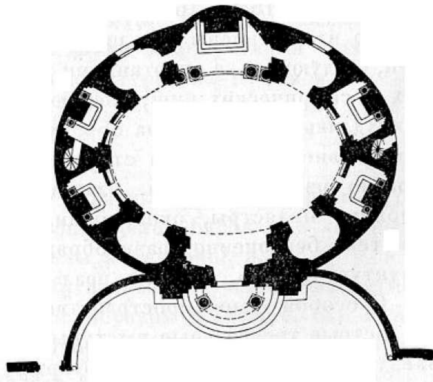
Церковь Сант Андреа аль Квиринале в Риме, (1658 г.) Арх. Л.Бернини.
