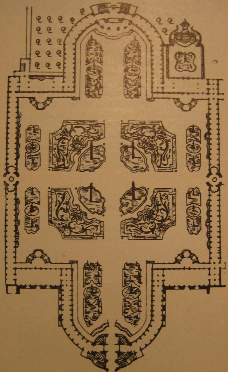
Цвингер в Дрездене, 1711—1722 г. Генеральный план
