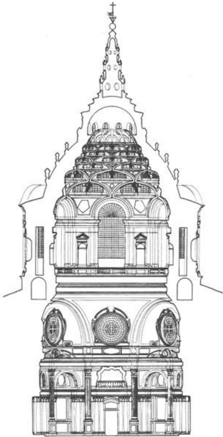
Капелла Сан – Синдоне в Турине. 1668 г. Арх. Гварино Гварини.
