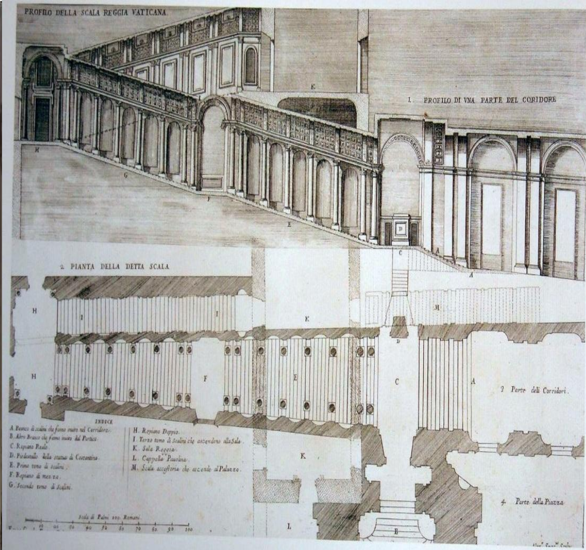
Королевская лестница («Скала реджа») в Ватикане. (1663 –1666 гг.)
