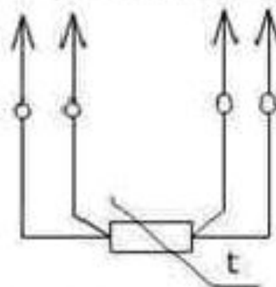
Четырехпроводная схема
