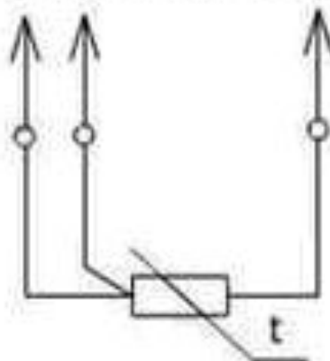
Трехпроводная схема
