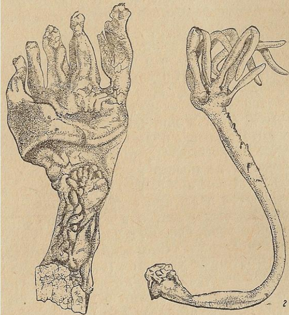
Рис. 45. 1 — Плодовое тело Fomes igniarius , выросшее при недостатке света; вид снизу; сохранено дорзовентральное строение, но край плодового тела разделяется как бы на 5 «пальцев»; 2 — Fomes applanatus , выросший в темноте; имеет радиальное строение, на вершине ветвится.
