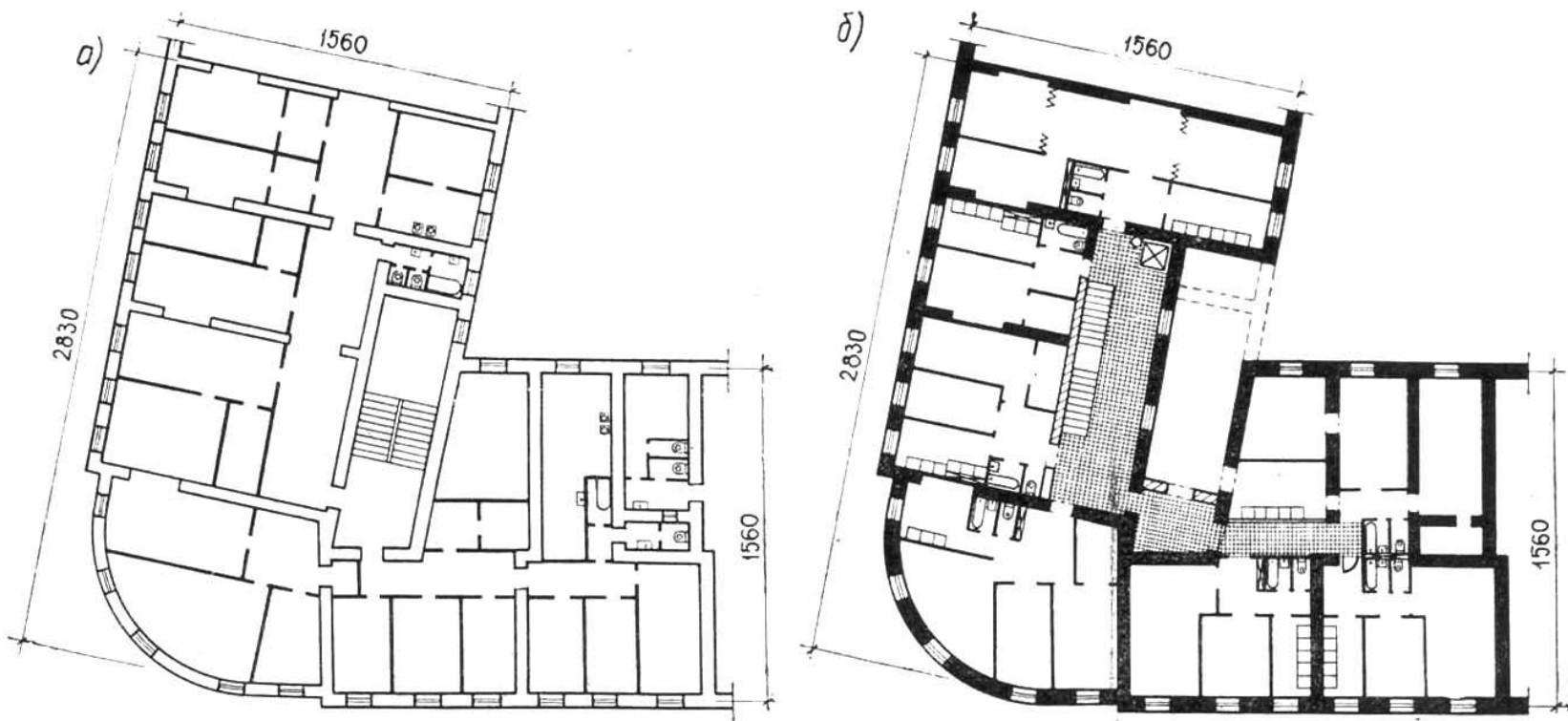
Пример реконструкции угловой секции широкого корпуса: a — до реконструкции; б — после реконструкции
