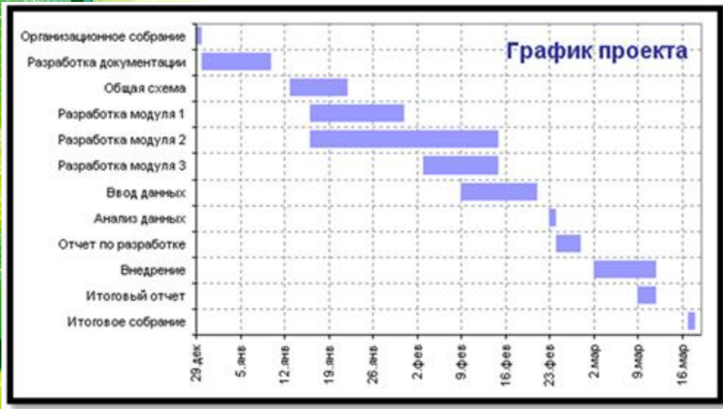
Диаграмма Ганта
