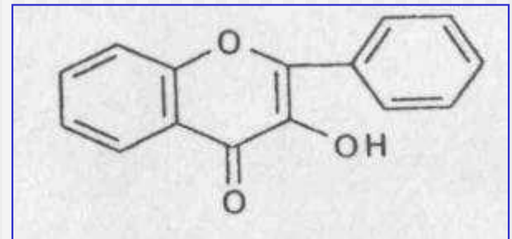
ФЛАВОНОЛ
