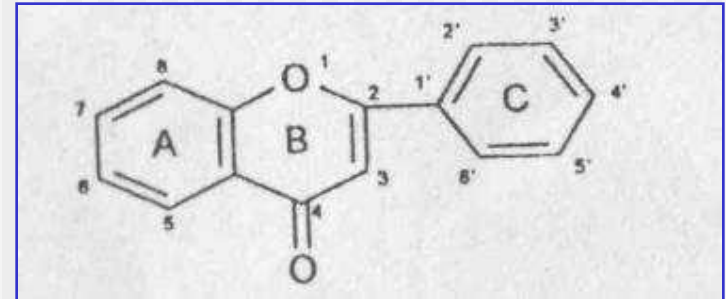
ФЛАВОН
