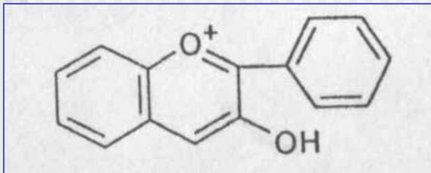
АНТОЦИАНИДИН
