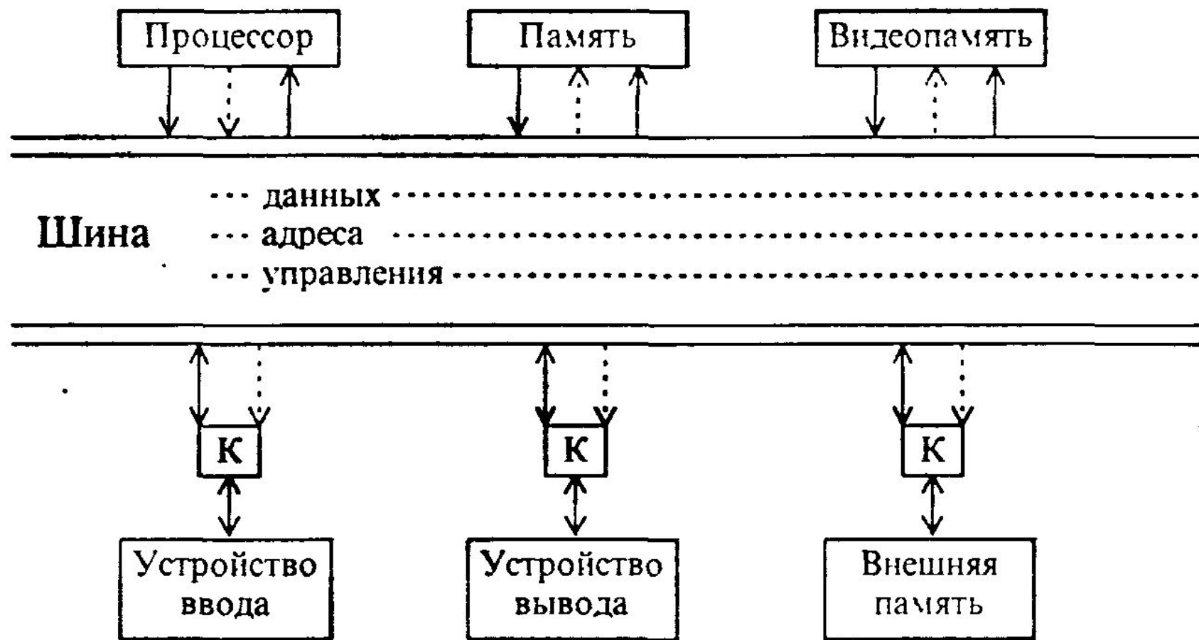
Шинная архитектура ЭВМ
