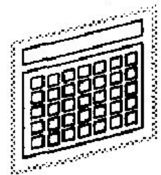
Электронная таблица
