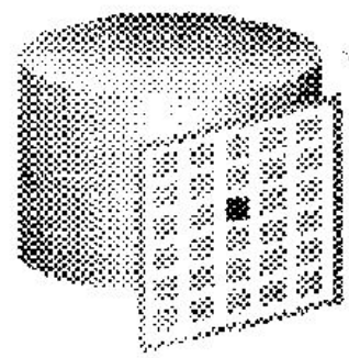
База данных
