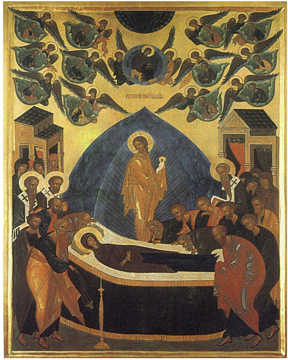
Одновременность событий
