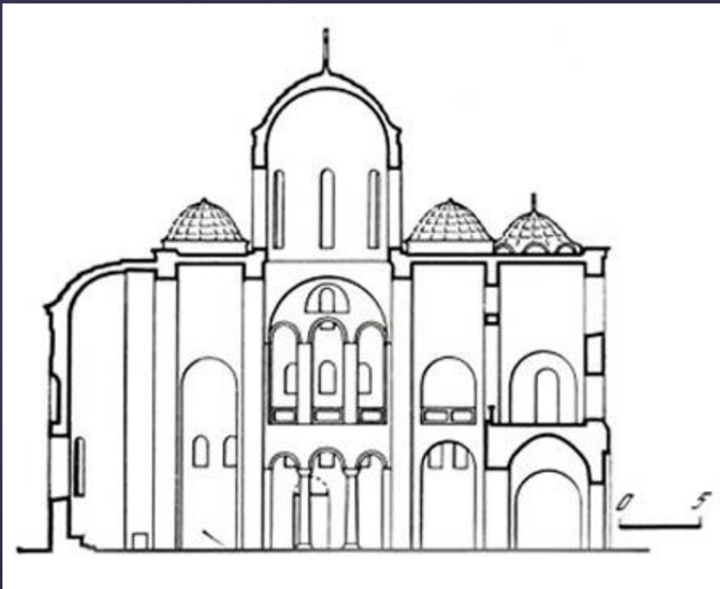
Спасо-Преображенский собор. Чернигов. 1030-1040-е годы. Схематический продольный разрез
