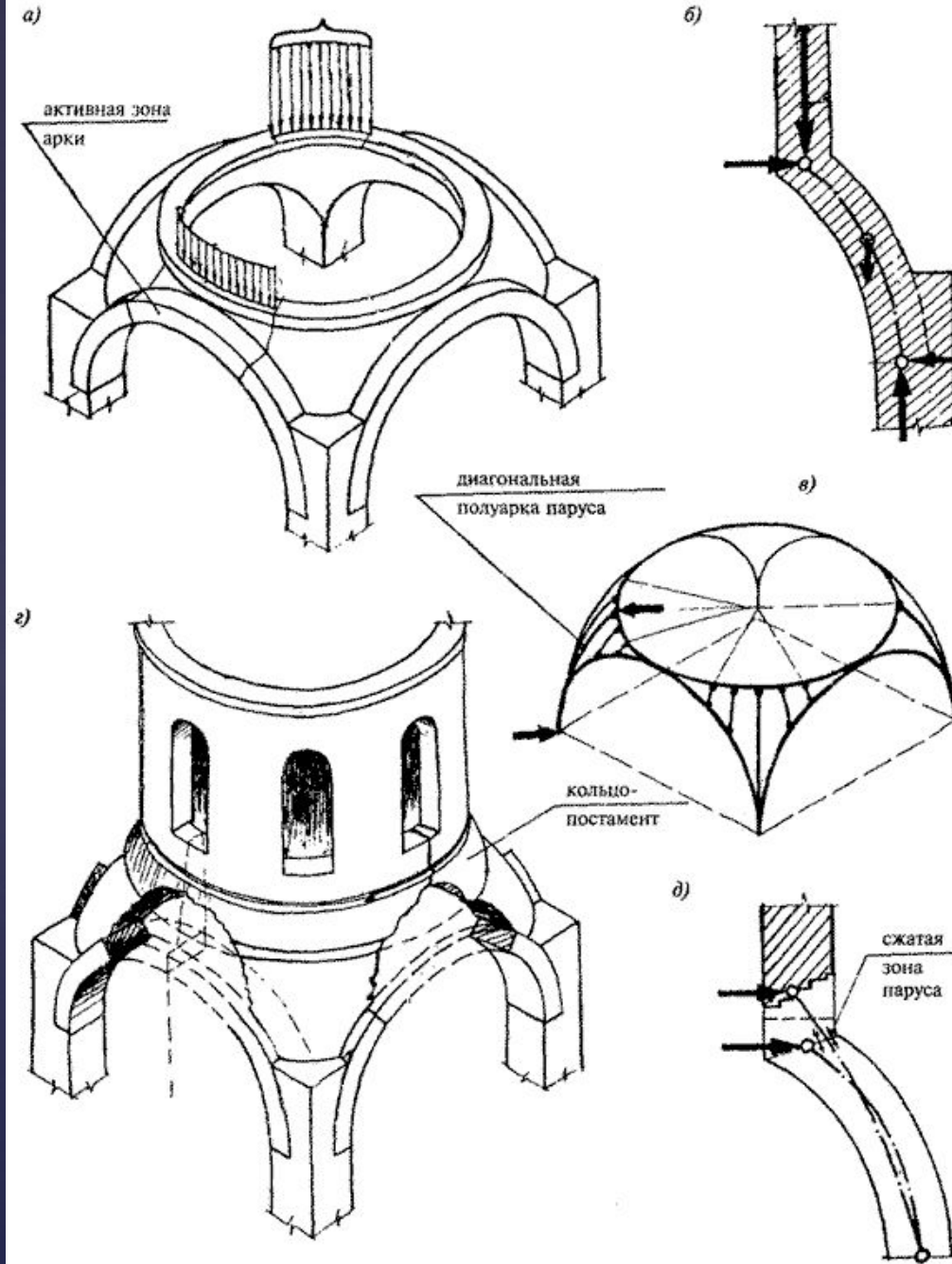
Схема крестово-купольного свода
