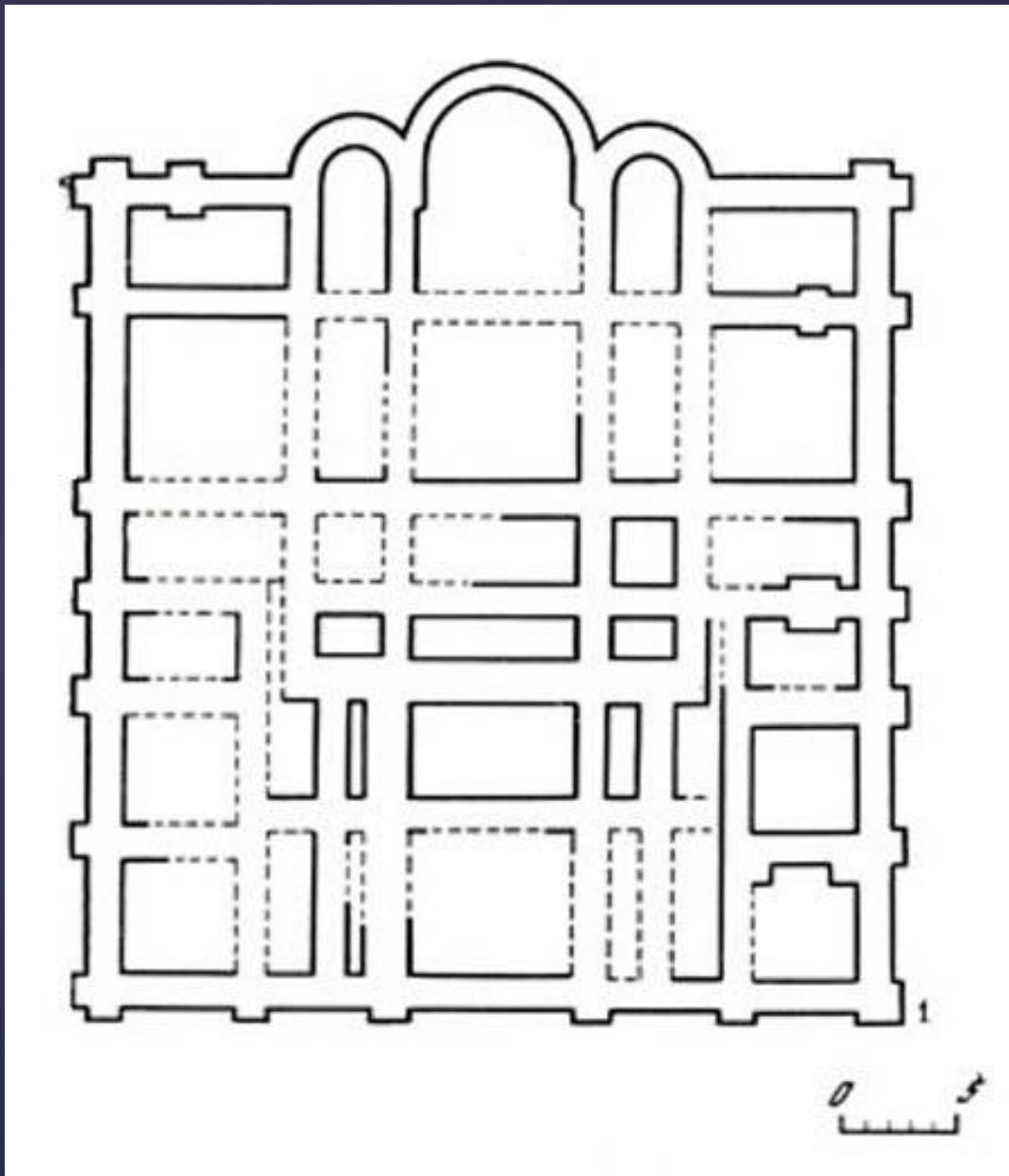
Киев. Десятинная церковь, 989-996 гг. План (по М К. Каргеру) и реконструкция Н. В. Холостенко
