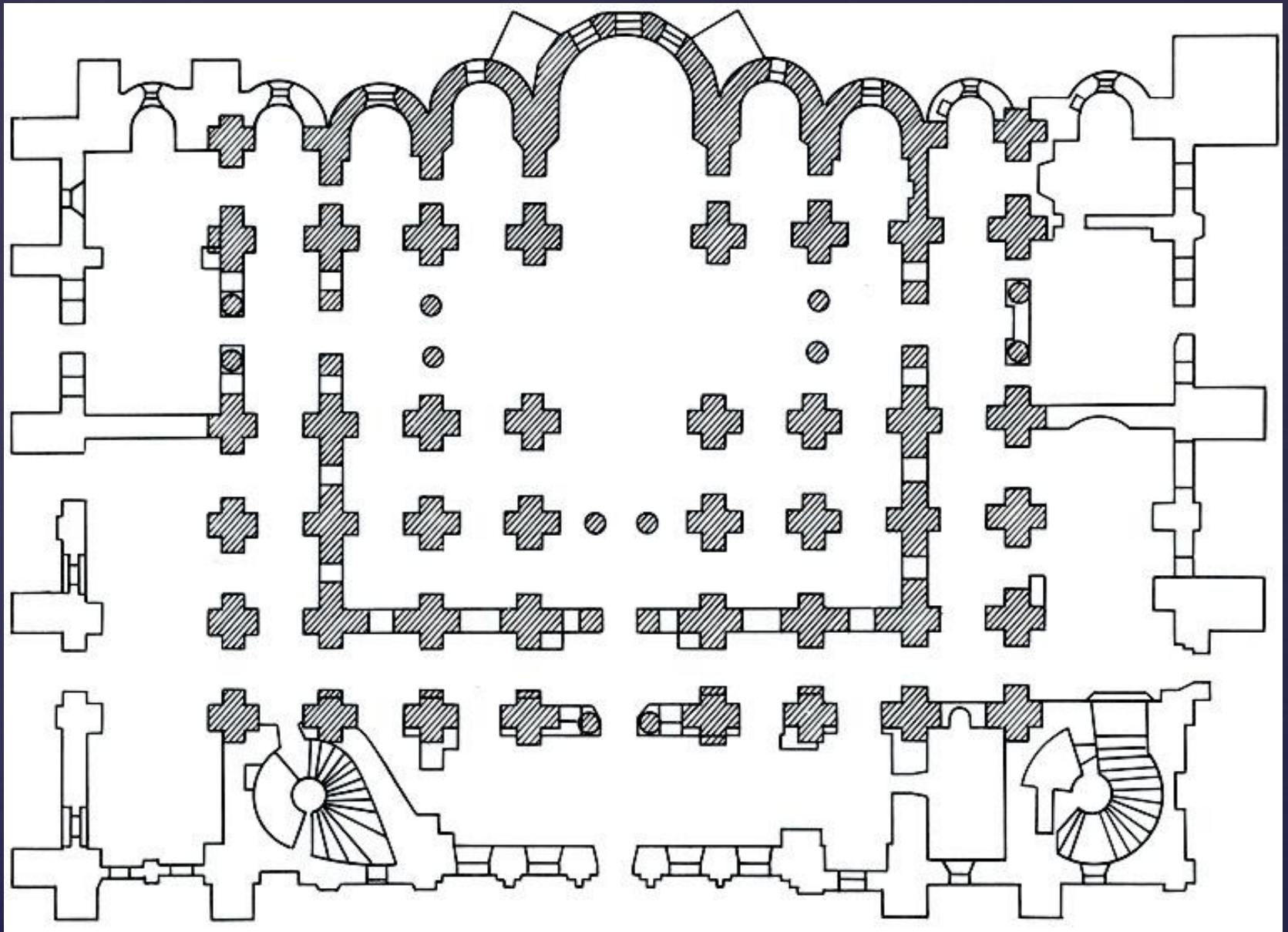
Софийский собор в Киеве. План.
