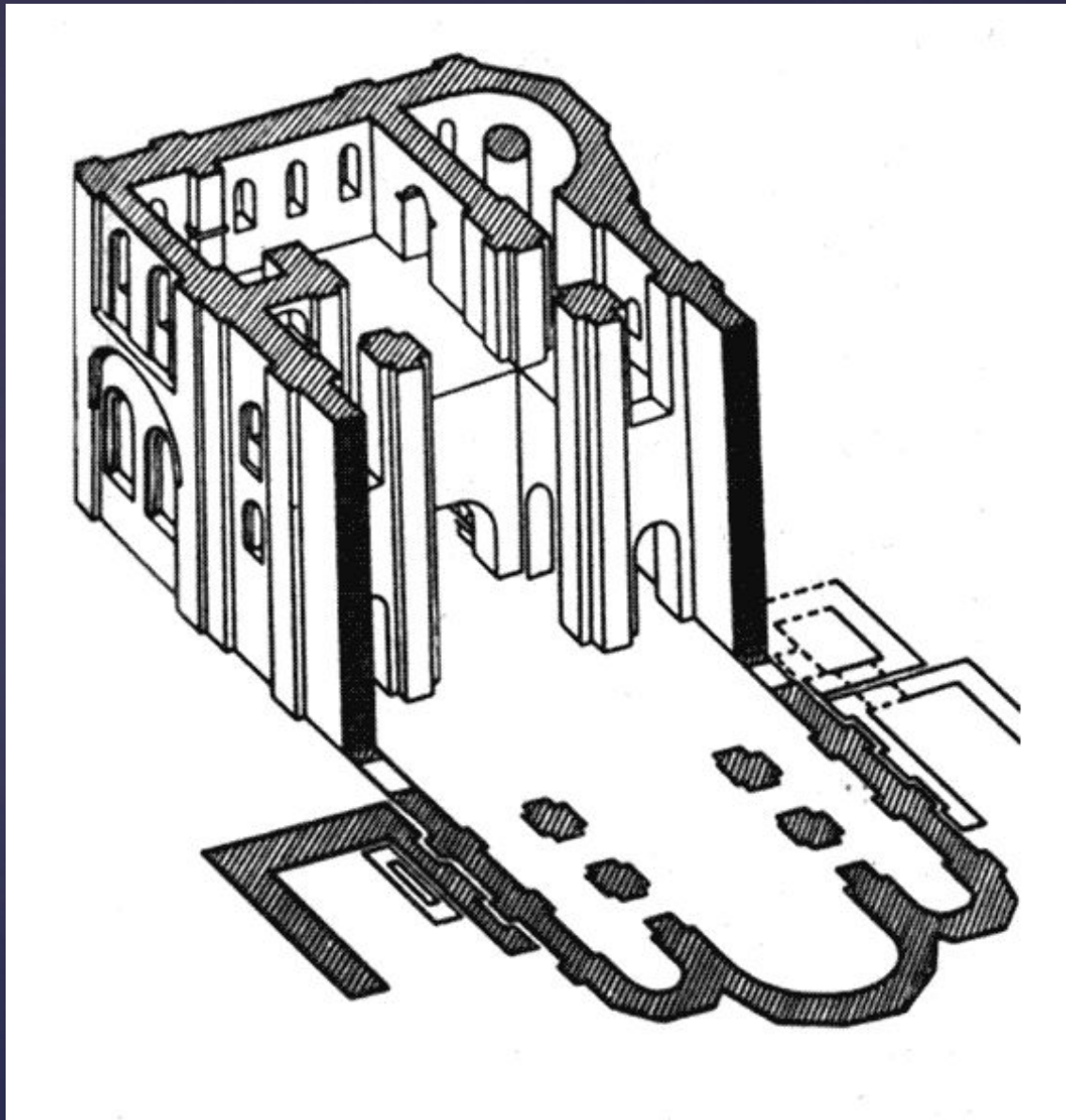
Михайловский собор Выдубецкого монастыря. 1070 - 1088. Аксонометрия. Чертеж М.Г. Каргера.
