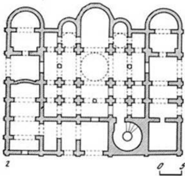
Планы пятинефных Софийских соборов в Киеве, Новгороде и Полоцке.
