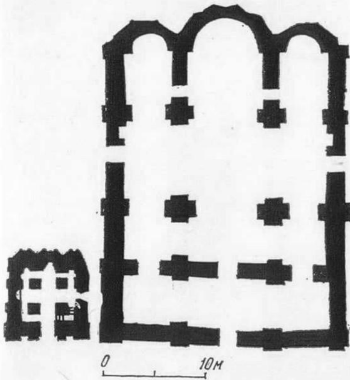
Успенский собор Печерского монастыря. План.
