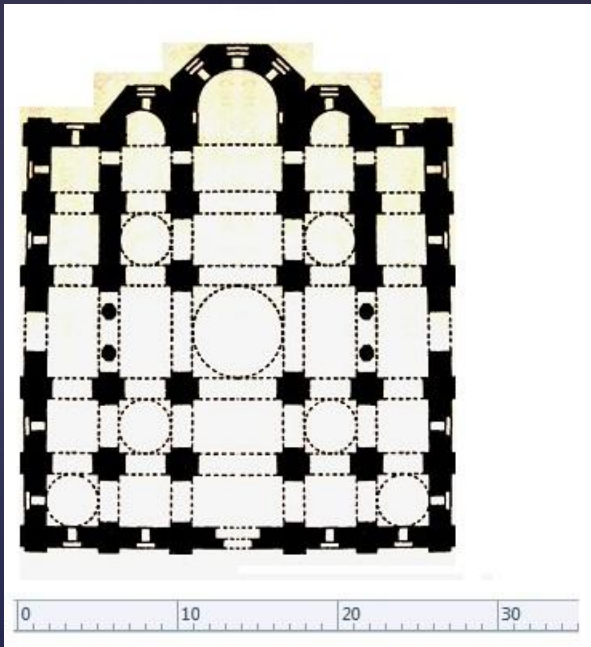
Софийский собор в Полоцке. План.
